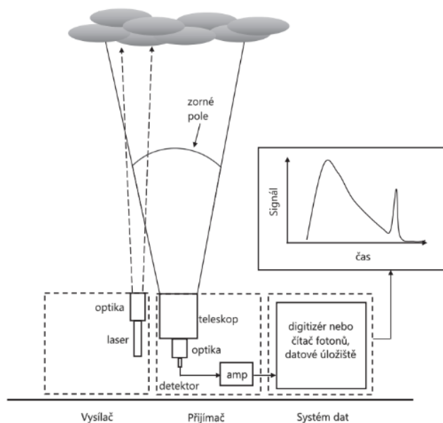
Obr. 3 Základní LiDARový systém (přeloženo)[40]
