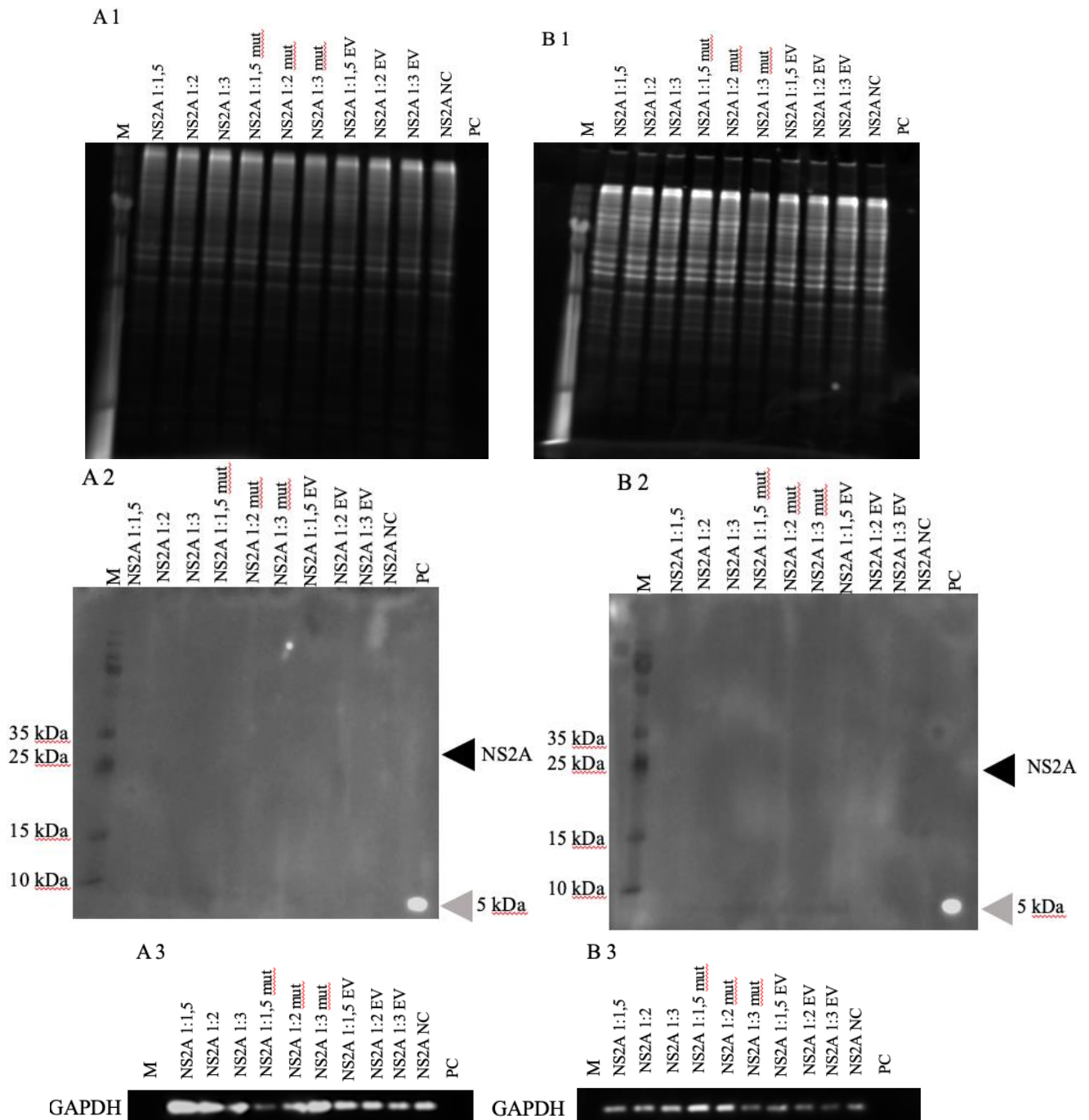
Obr.14: Optimalizace podmínek detekce proteinu NS2A v transfekovaných buňkách pomocí imunoblodu. Vizualizace signálu TCE v redukujících (A1) a neredukujících (B1) podmínkách po elektroforetické separaci, detekce proteinu NS2A – vzorky v redukujících (A2) a neredukujících (B2) podmínkách pomocí imunoblodu, detekce proteinu GAPDH v redukujících (A3) a neredukujících (B3) podmínkách. Zkratky: M – velikostní standard, NS2A – protein NS2A wild type (~25 kDa), NS2A mut – protein NS2A mutovaný (~25 kDa), NS2A EV – kontrolní vektor, NS2A NC – negativní kontrola, PC – pozitivní kontrola, 1:1,5 – transfekční poměr (plasmid: transf. reagens), 1:2 - transfekční poměr (plasmid: transf. reagens), 1:3 - transfekční poměr (plasmid: transf. reagens), černá šipka – očekávaný signál proteinu NS2A, šedá šipka – signál NS2Apep (5 kDa) PC.
