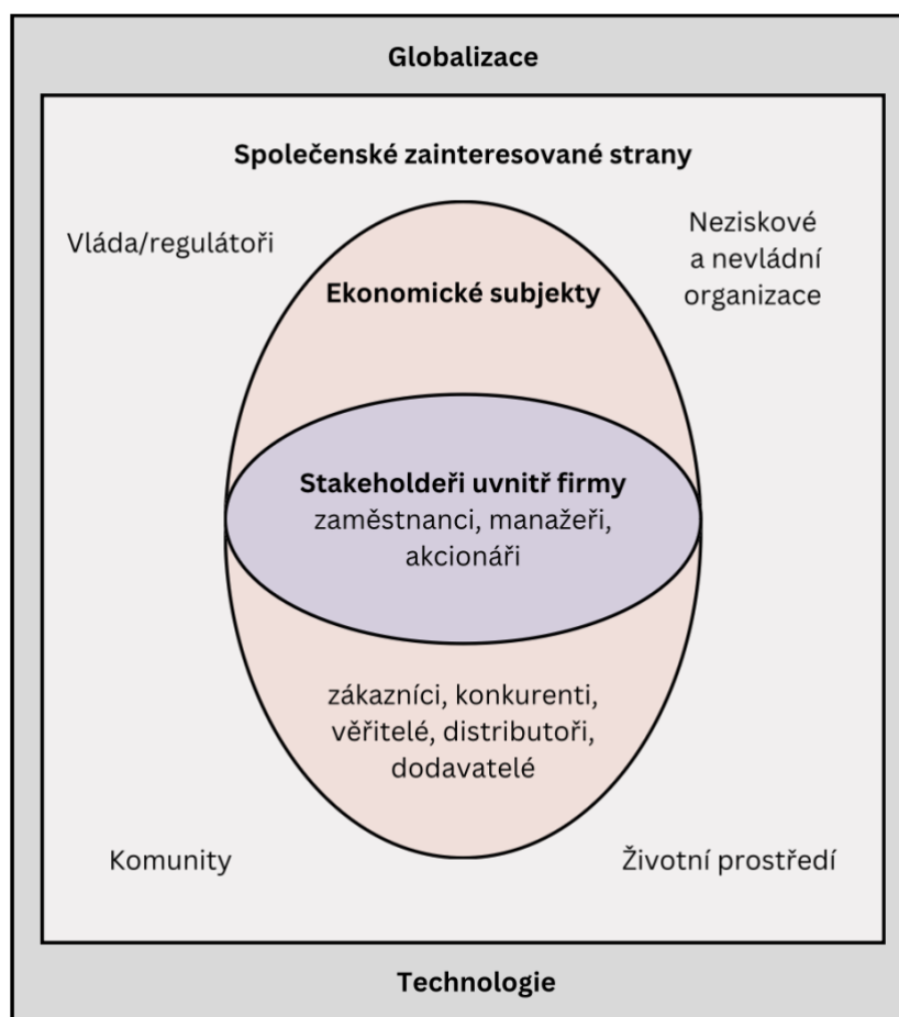
Obrázek 35: Stakeholder model
