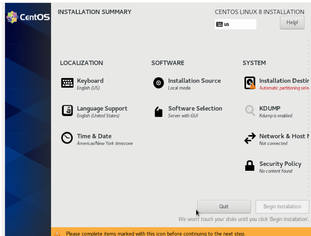
Obrázek 2.3 Instalace CentOS
