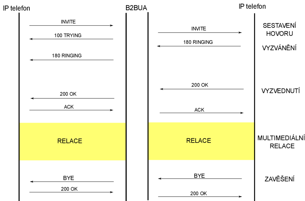
Obrázek 1.3 Komunikace s využitím B2BUA
