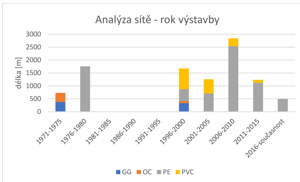
Obrázek 24: Skutečná síť – rok výstavby
