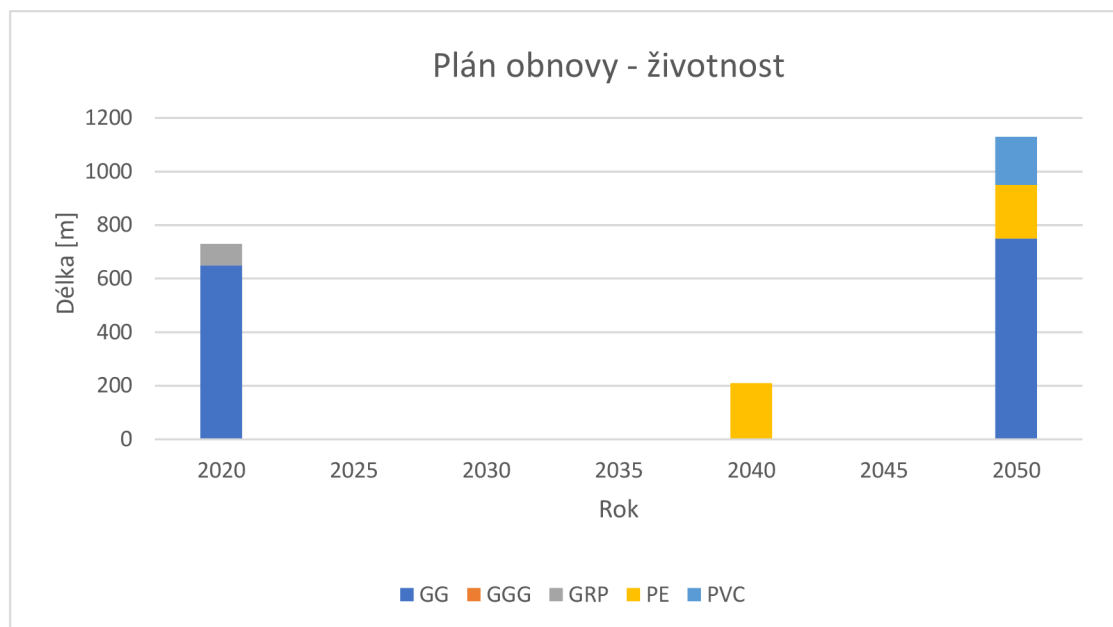
Obrázek 21: Plán obnovy na základě životnosti potrubí
