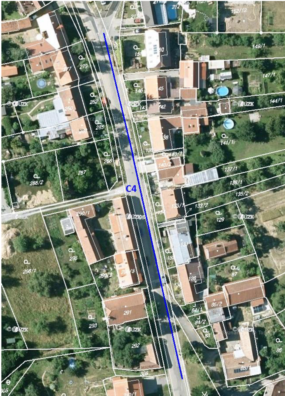
Obrázek 26: Poloha vodovodního řadu C4 v katastrální mapě [15]
