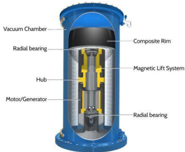
Obr. 3 Setrvačnicková baterie [84]
