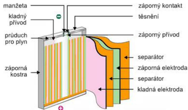
Obr. 6 Řez lithiovým akumulátorem [24]
