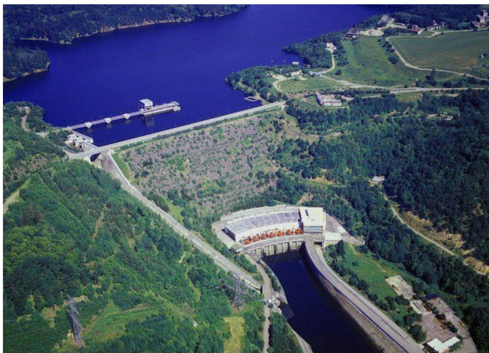
Obr. 10 Přečerpávací vodní elektrárna Dalešice [12]
