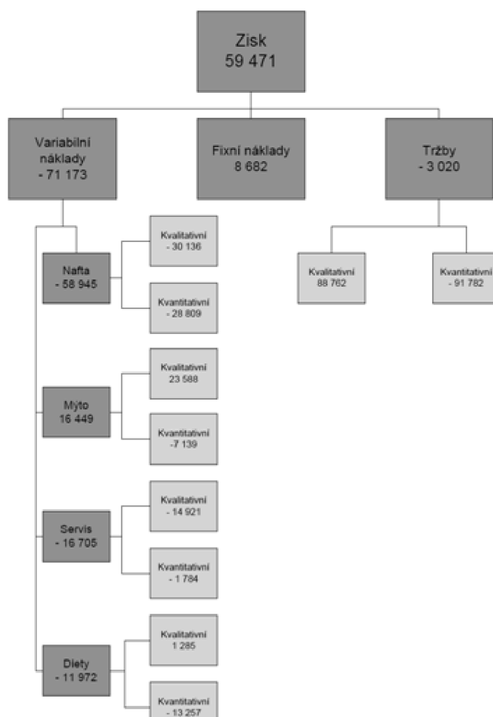
Obrázek č. 7: Rozklad celkové odchylky voziidla do 12 tun v roce 2017 na jednotlivé vlivy (v Kč). Vlastní zpracování dle (17).
