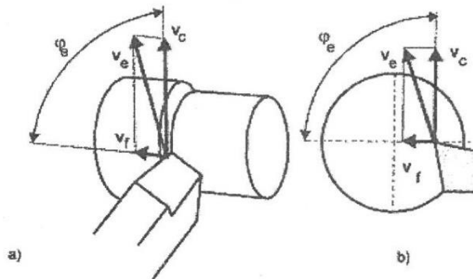
Obr. 4.7 Směry vektorů hlavního a vedlejšího pohybu při válcovém a čelním soustružení [2].
