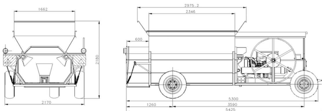
Obr. 1.9 Pracovní rozměry kompostovací lis CM 1,5.
