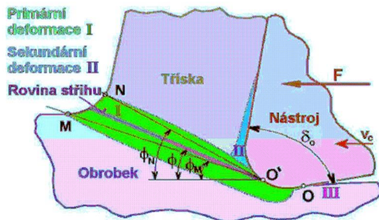
Obr. 4.3 Oblasti plastických deformací procesu řezání [7].
