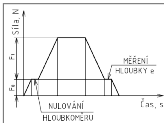
Obr. 6 Časový průběh zkoušky Rockwell [6]
