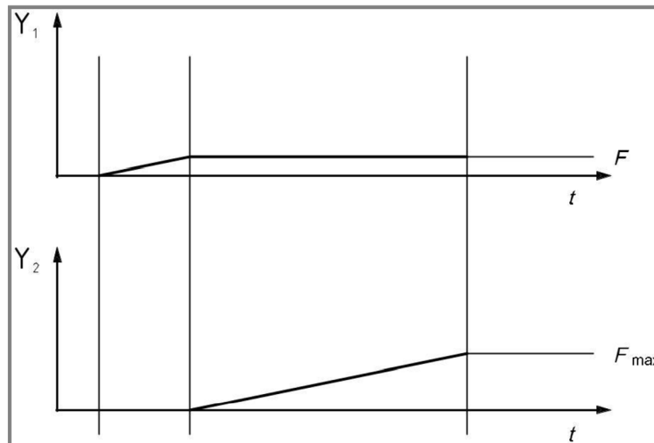
Obr. 19 Závislost zatížení a posuvu na čase, CFST [7]
