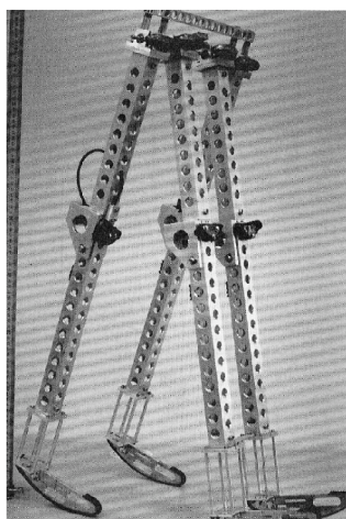
(a) Dvojrzmerný pasívny chodec [11]
