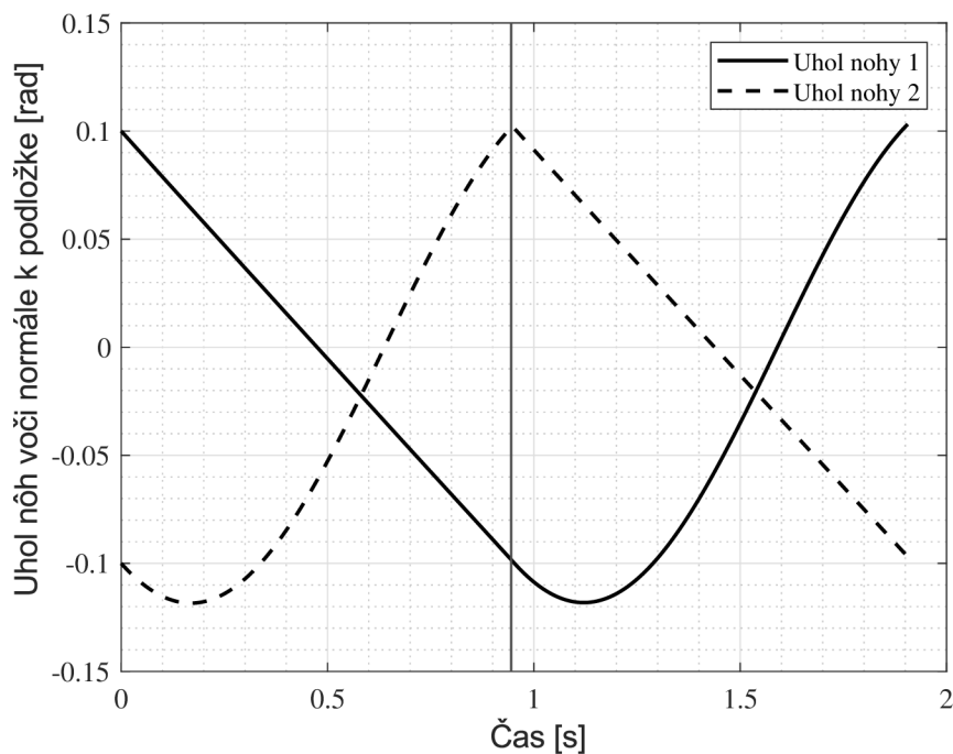
Obrázok 3.9: Priebeh uhlov nôh voči normále k podložke pri podmienkach chôdze s krátkou periódou získaný zo simulácie v Simscape Multibody. l = 1 m, m_T = 50 kg, m_L = 0,1 kg, m_F = 0,1 kg, \alpha_i = 0,1 rad, g = 9,81 m s -2
