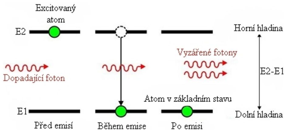
Obr. 4 Princip vzniku stimulované emise [41].
