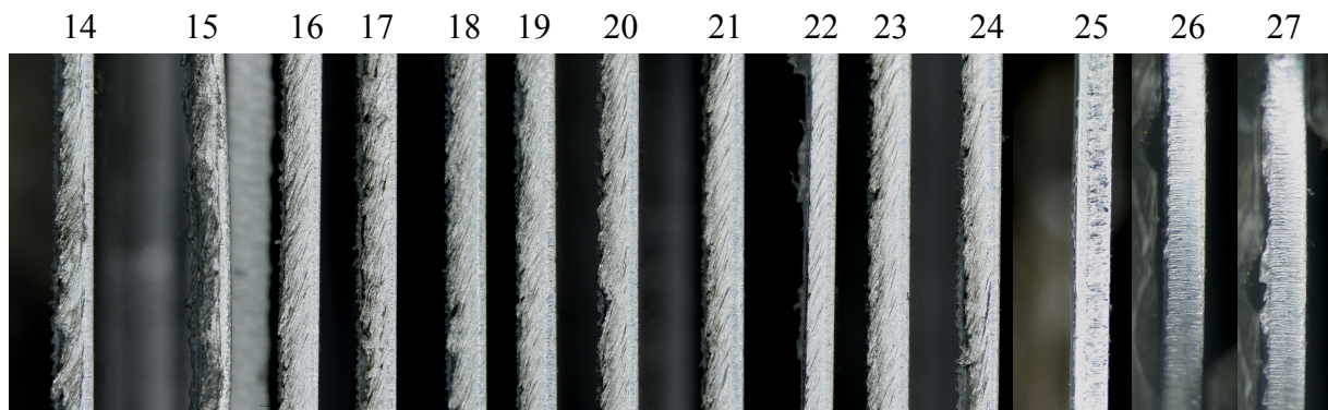
Obr. 53a Velikost otřepů vzorků s fólií umístěnou na spodní straně řezu.
