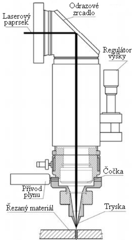
Obr. 14 Řezací hlavice [1].
