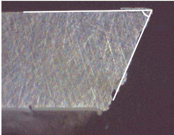
Obr. 60 Vzorek WaterJet.
