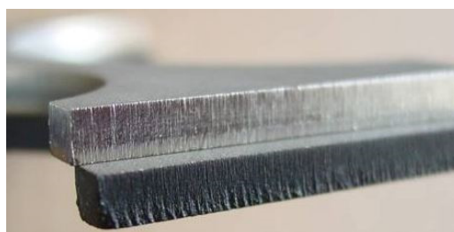
Obr. 17 Řezná hrana ovlivněná typem použitého řezného plynu [1].
