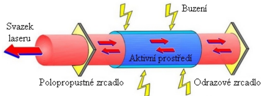
Obr. 5 Konstrukce laseru [41].
