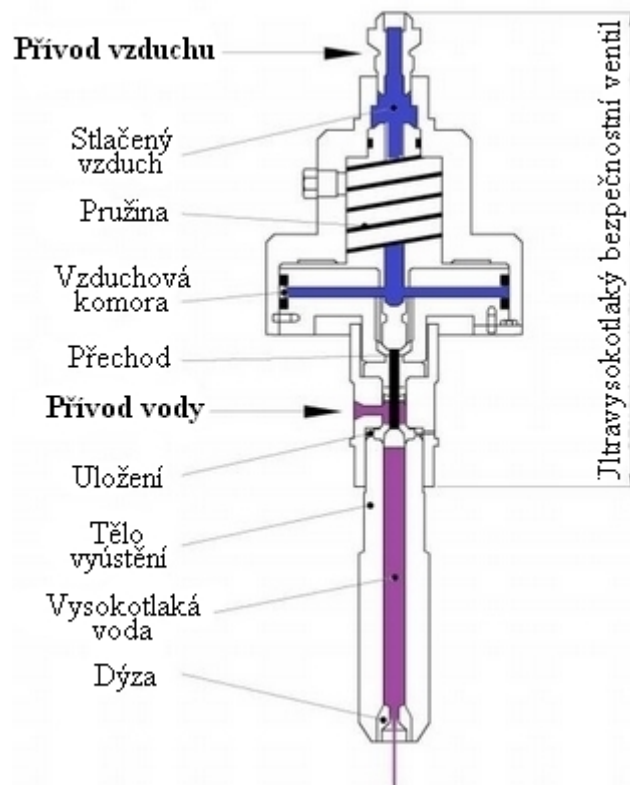
Obr. 28 Tryska WJM [45].
