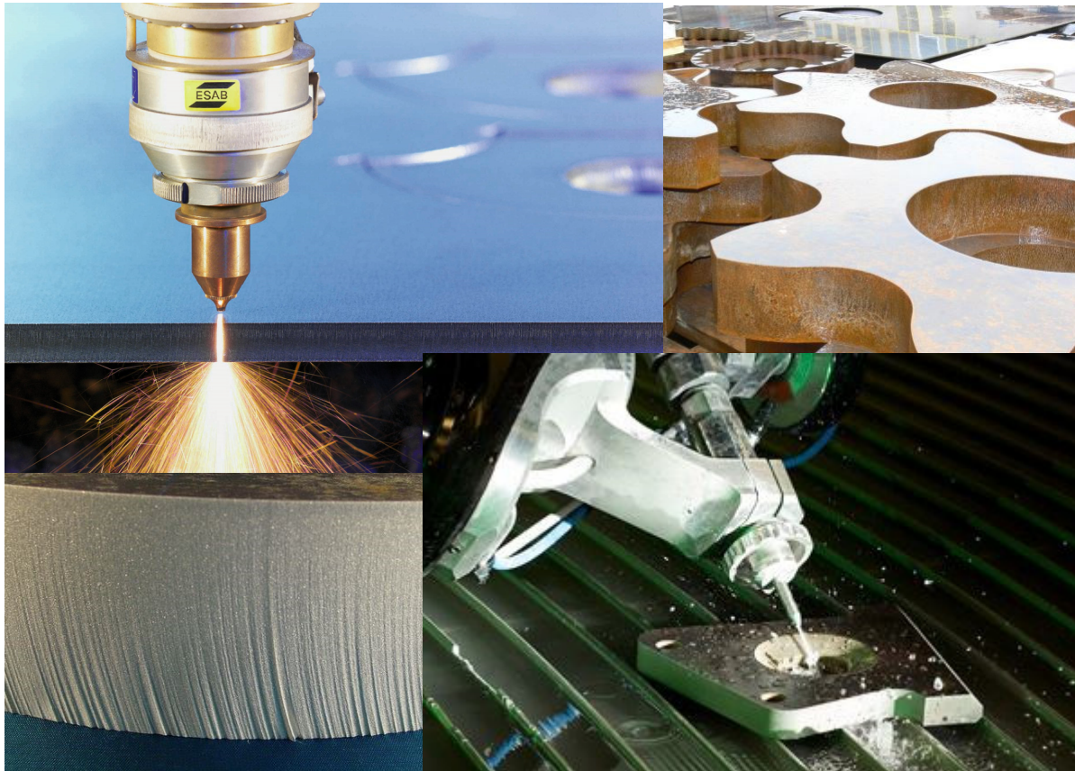
Obr. 1 Příklady řezání vodním paprskem a laserem [13], [24], [55].
