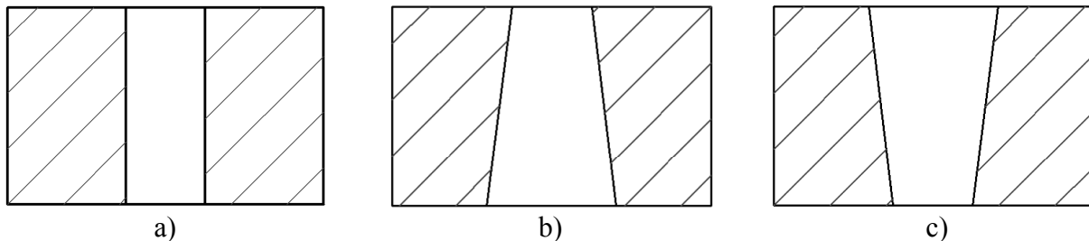
Obr. 33 Odchylny kolmosti.
