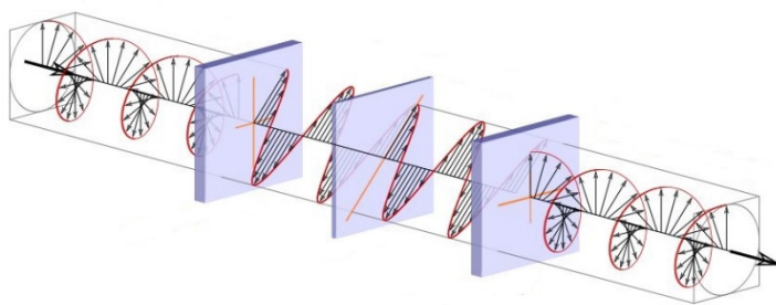
Obr. 12 Polarizace [1].
