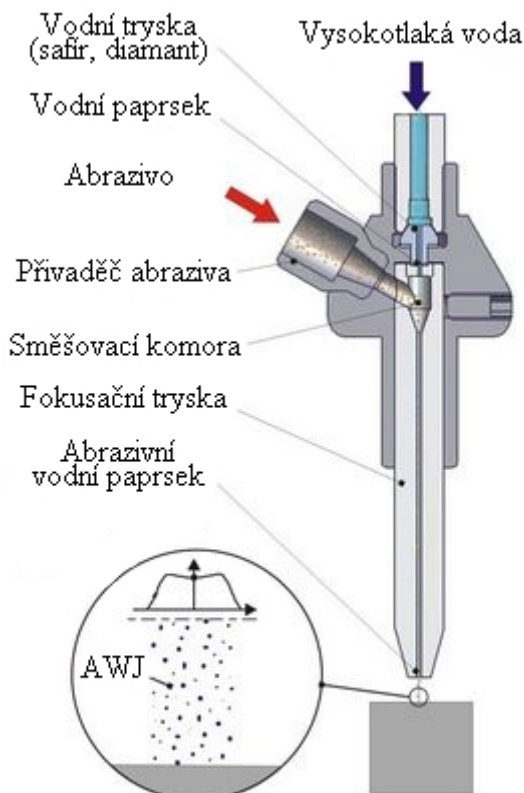
Obr. 29 Tryska AWJ [26].
