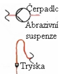
Obr. 30 Systém přímého vstřikování [36].
