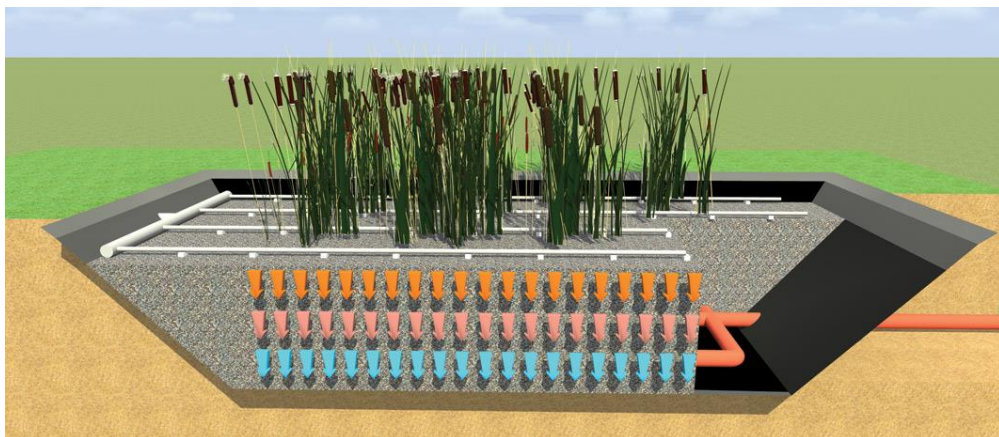
Obr. 18 Schéma vertikálního kořenového filtru (zdroj: Michla Křiška)
