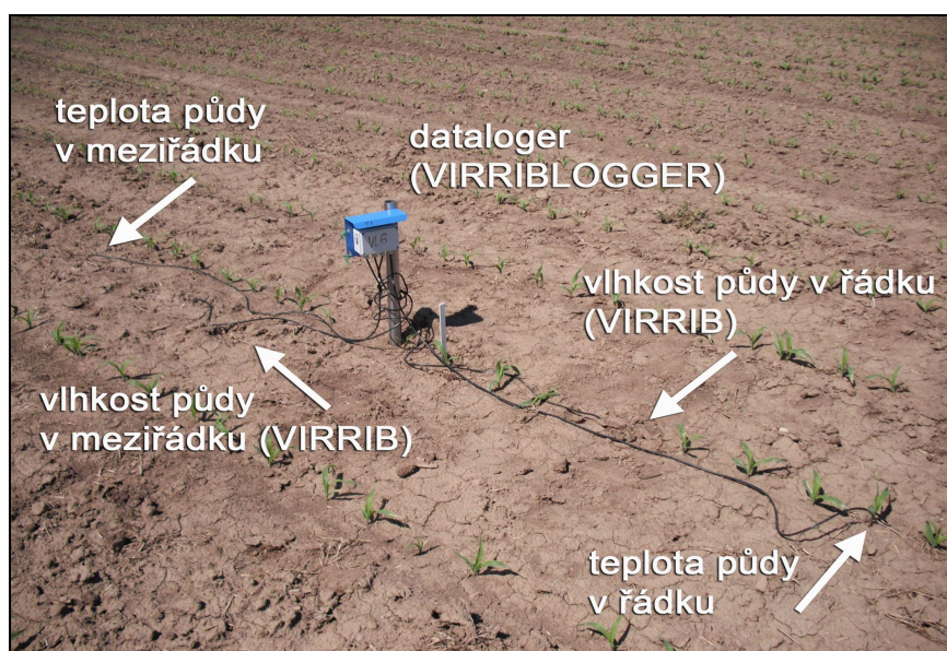
Obrázek 6 Popis umístění snímače půdní vlhkosti VIRRIB (zdroj: archiv autora)
