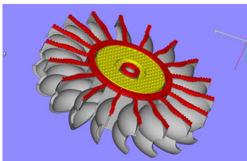
Obrázek 34 - Podpory u tisku SLA
