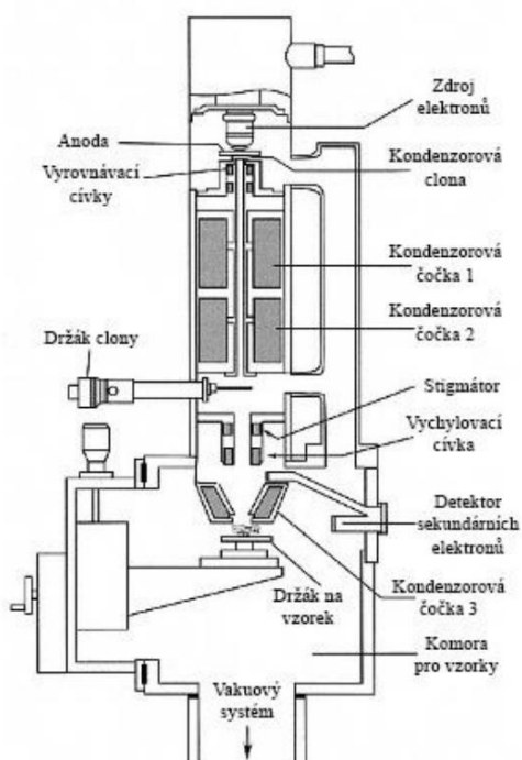
Obrázek 28 - Schéma SEM
