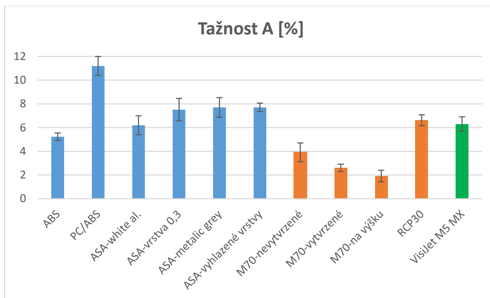
Graf 4 - Tažnost materiálů 3D tisku
