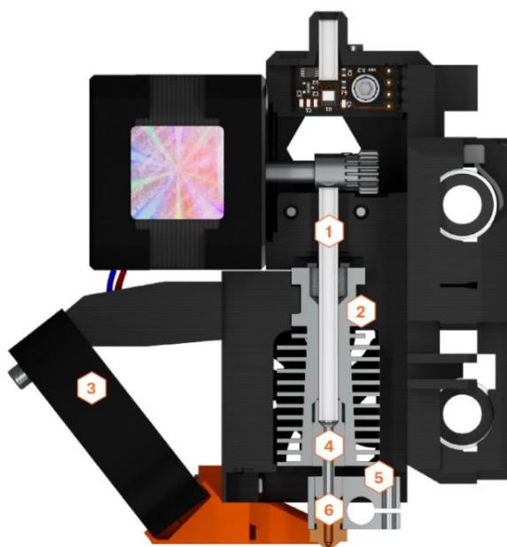
Obrázek 6 - Extrudér. 1-teflonová trubice, 2-chladič, 3-tiskový ventilátor, 4-izolátor, 5-ohřívací blok, 6-tryska (3)
