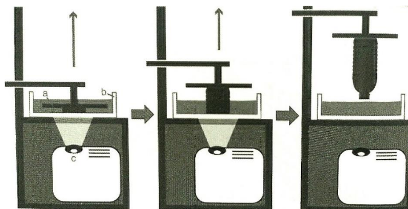
Obrázek 10 - Proces tisku SLA tiskárny
