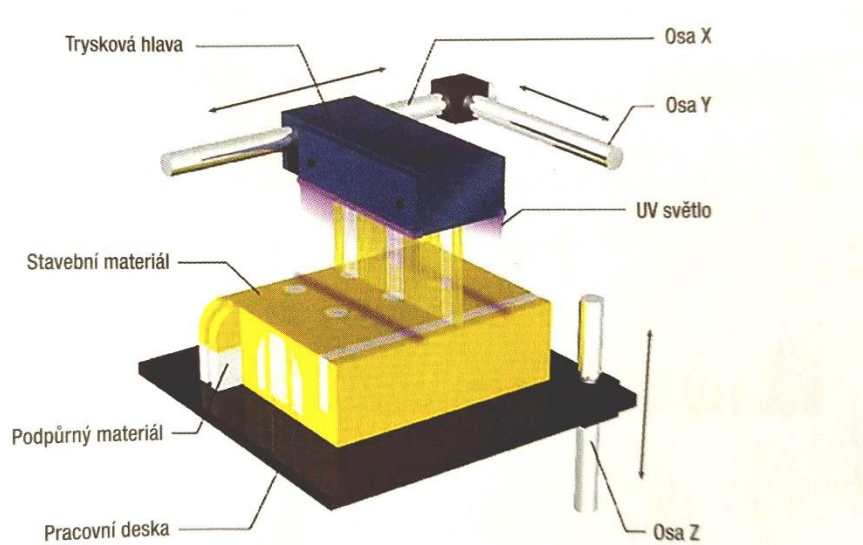
Obrázek 13 - Schéma MJP tisku (17)
