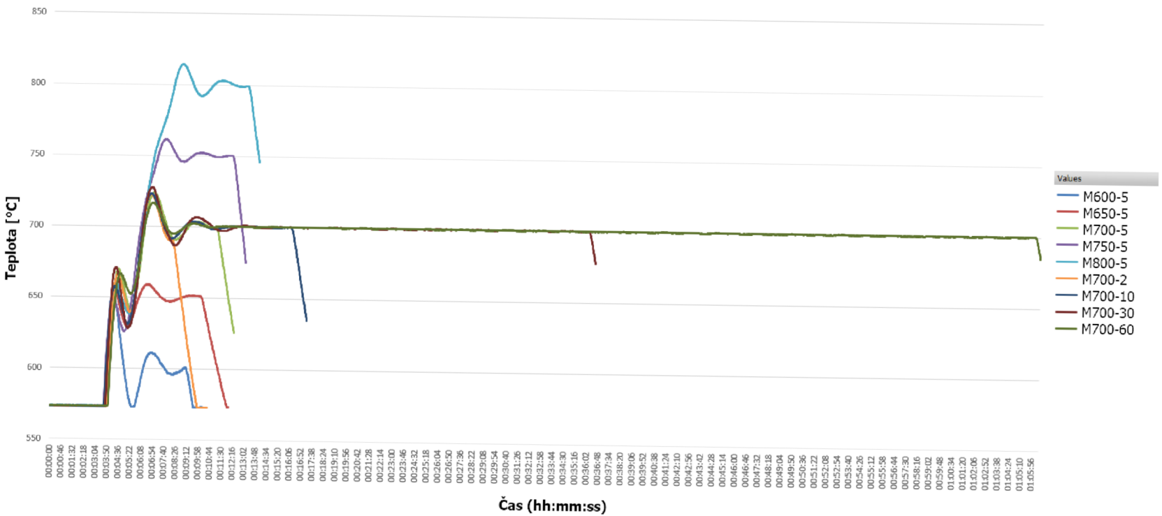
Obrázok P1.1: Priebeh teplôt spekania v zariadení SPS u rôznych vzoriek SiO 2 -mletého
