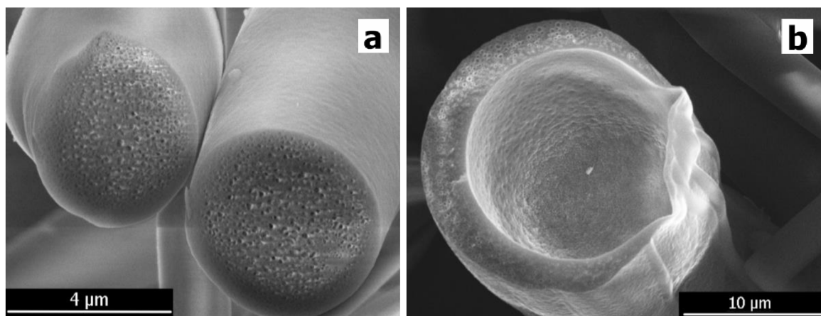
Obrázok 4.2: Detaily na rez vláknami \text{SiO}_2 zobrazujúce prítomnosť mezopórov (a – v celom objeme; b – na okrajoch a vnútornom povrchu)
