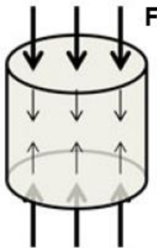
Obrázok 4.5: Znáznornenie silového pôsobenia počas kompresného testu [62]
