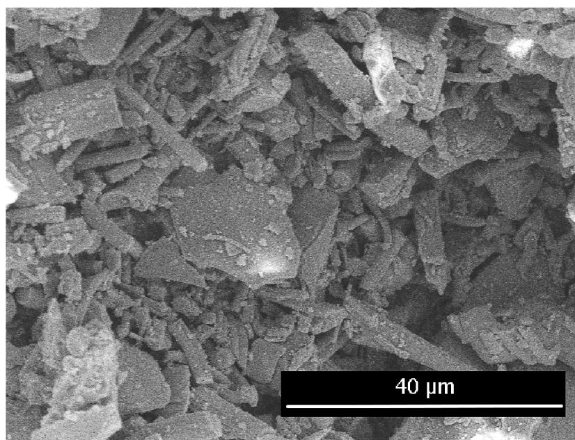
Obrázok 4.3: Pohľad na nespracované, ale pomleté vlákna \text{SiO}_2 pomocou SEM
