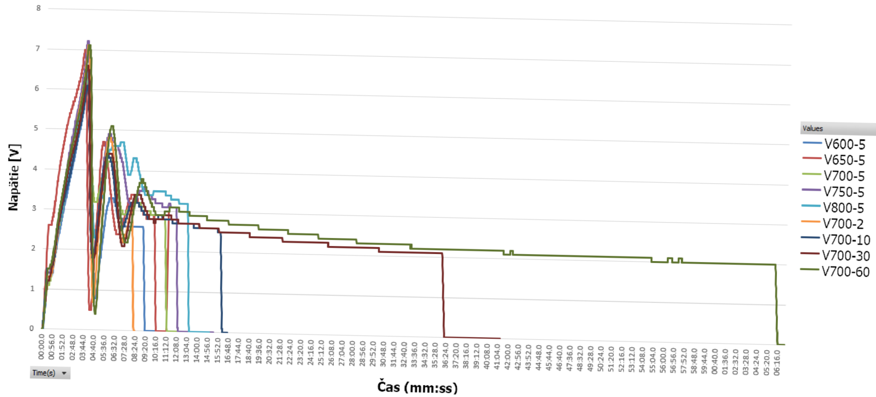
Obrázok P1.2: Priebeh napätia pri spekaniach v zariadení SPS u rôznych vzoriek SiO 2 -vlákien
