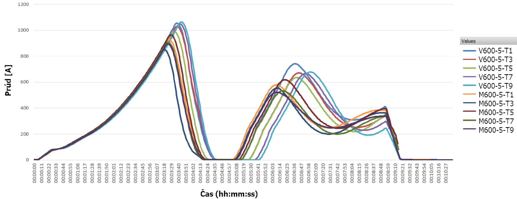
Obrázok P1.3: Priebeh elektrického prúdu pri spekaniach v zariadení SPS, porovnanie vzoriek \text{SiO}_2 -vlákien a \text{SiO}_2 -mletého (hodnoty vzoriek použitých na mechanické testovanie)
