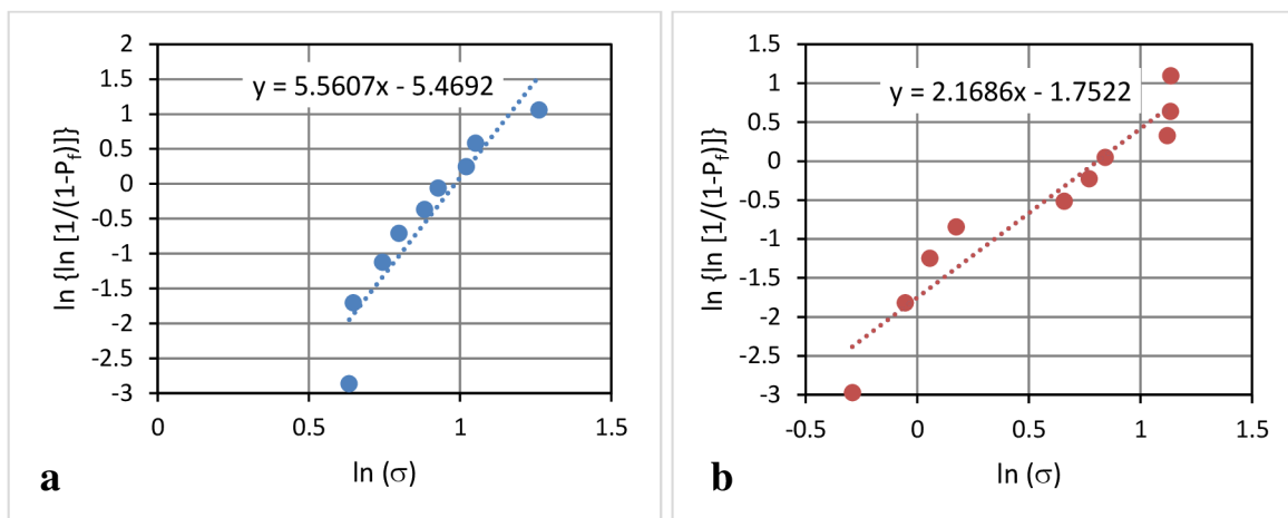
Obrázok 5.8: Grafy určujúce Weibullov modul (a – \text{SiO}_2 -vlákna, b – \text{SiO}_2 -mleté)
