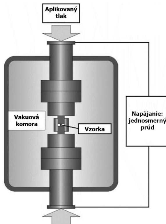
Obrázok 3.10 Schéma zariadenia SPS [46]
