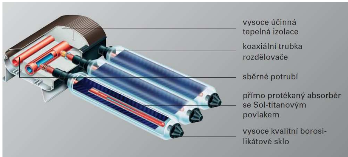
Obr. 2.2 Vakuové trubice s přímo protékaným absorbérem. [6]
