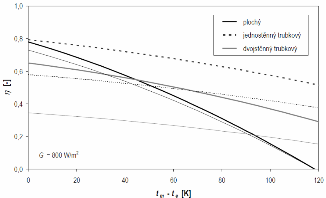
Obr. 2.4 Příklad křivek účinnosti jednotlivých typů kolektorů při ozáření 800 \text{W/m}^2 . [4]
