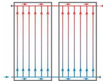
Obr. 3.6 Schéma zapojení kolektoru se sběrným potrubím v horní i spodní části [11]
