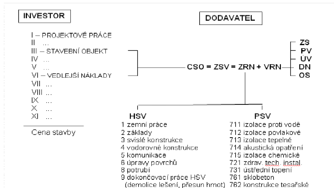
Obrázek 2 - Struktura rozpočtu [4]
