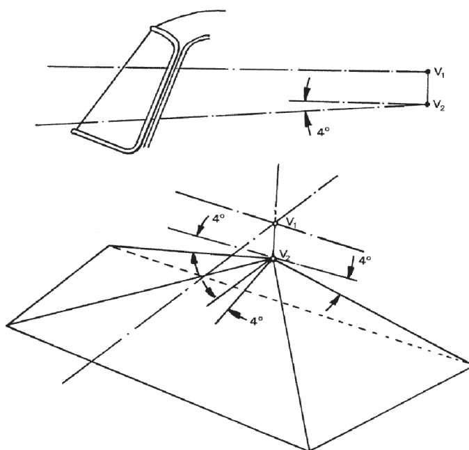
Obrázek 25: Zakrytí pole výhledu v úhlu 180^\circ
