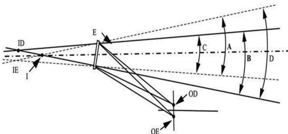
Obrázek 7: Ambinokulární vidění
