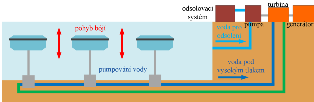
Obr. 4.6: technologie CETO
