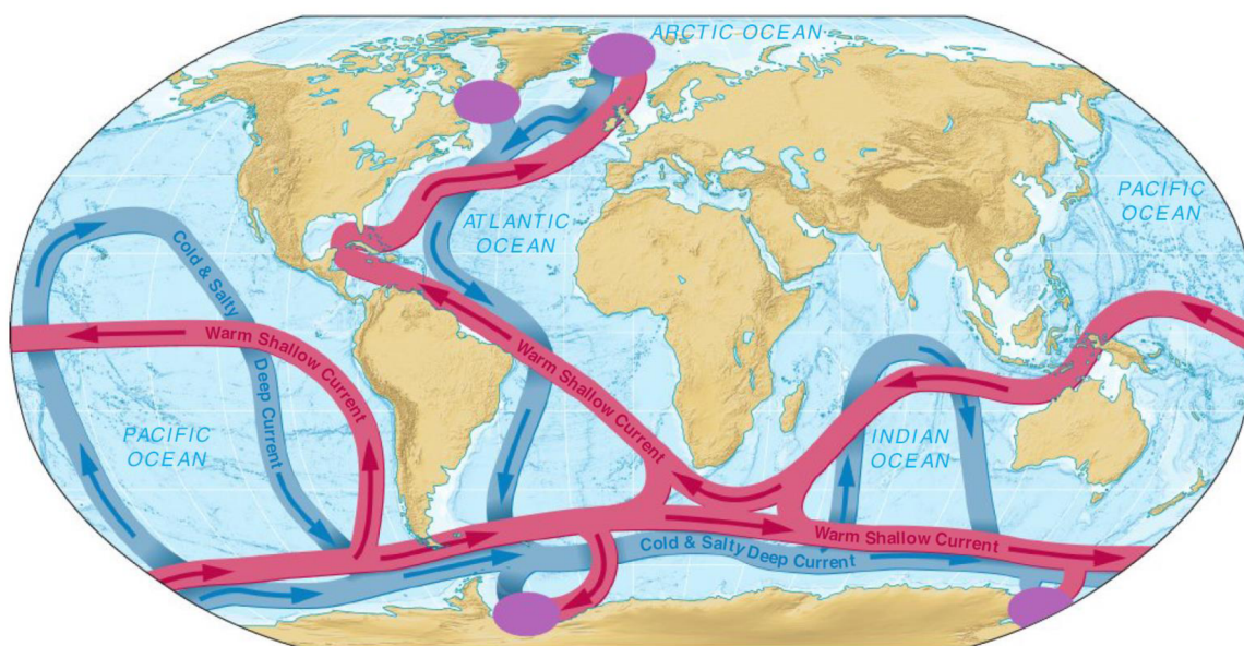
Obr. 3.3: Idealizovaná schématická mapa termohalinní cirkulace (převzato z [2])
