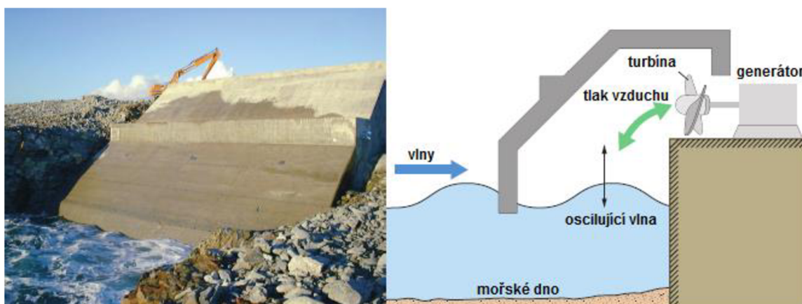
Obr. 4.3: Elektrárna typu LIMPET (převzato z [2])
