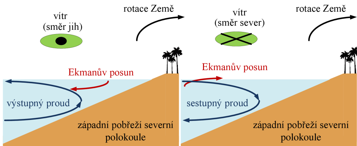
Obr. 3.4: Pobřežní výstupné a sestupné proudy
