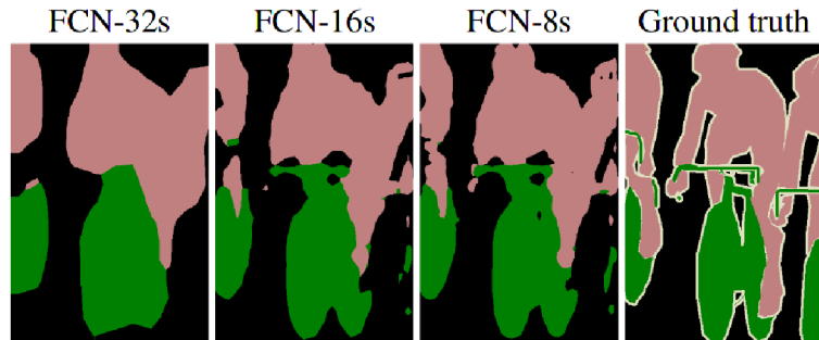
Obrázek 4.2: Porovnání výsledků kroků 8, 16 a 32 pixelů a originálního ground truth. Převzato z [40].
