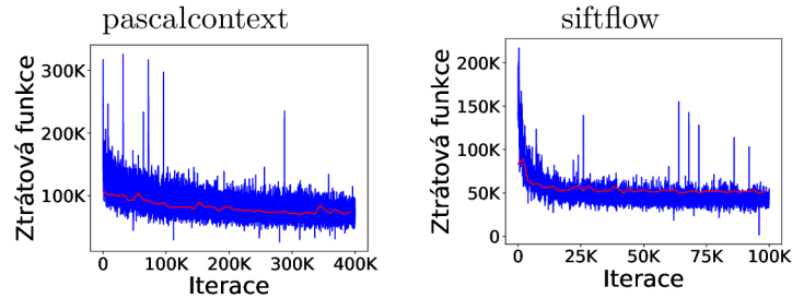
Obrázek 6.4: Graf ztrátové funkce prvního kroku dotrénování modelů pascalcontext-fcn8s a siftflow-fcn8s na datové sadě s neredukovaným počtem tříd. Graf obsahuje hodnoty ztrátové funkce na trénovací množině (modrá barva) a na validační množině (červená barva).
