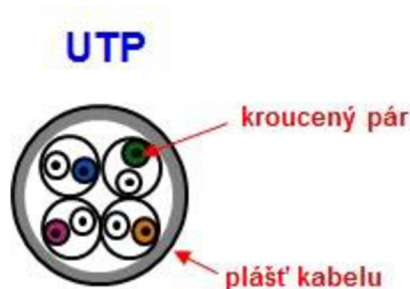
Obrázek 11: UTP – nestíněný párový kabel. (Zdroj: ONDRÁK, V. Počítačové sítě – Reálná přenosová prostředí . Přednáška, s. 9)
