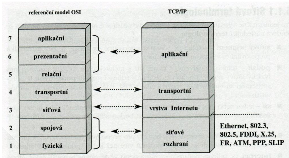
Obrázek 6: Porovnání architektury TCP/IP s referenčním modelem OSI. (Zdroj: PUŽMANOVÁ, R. Moderní komunikační síť od A do Z , s. 246)
