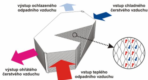
Obr. 3.2: Funkční schéma protiproudého rekuperačního výměníku [10]
