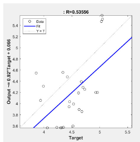
Obrázok 12 Regresia testovania pri nastavení \max\_fail=30
