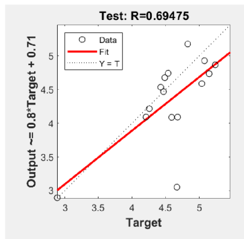
Obrázok 11 Regresia testovania pri nastavení \mu=1
