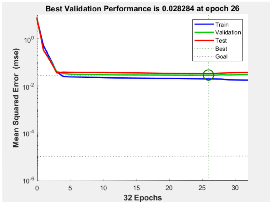
Obrázok 6 Graf procesu učenia
