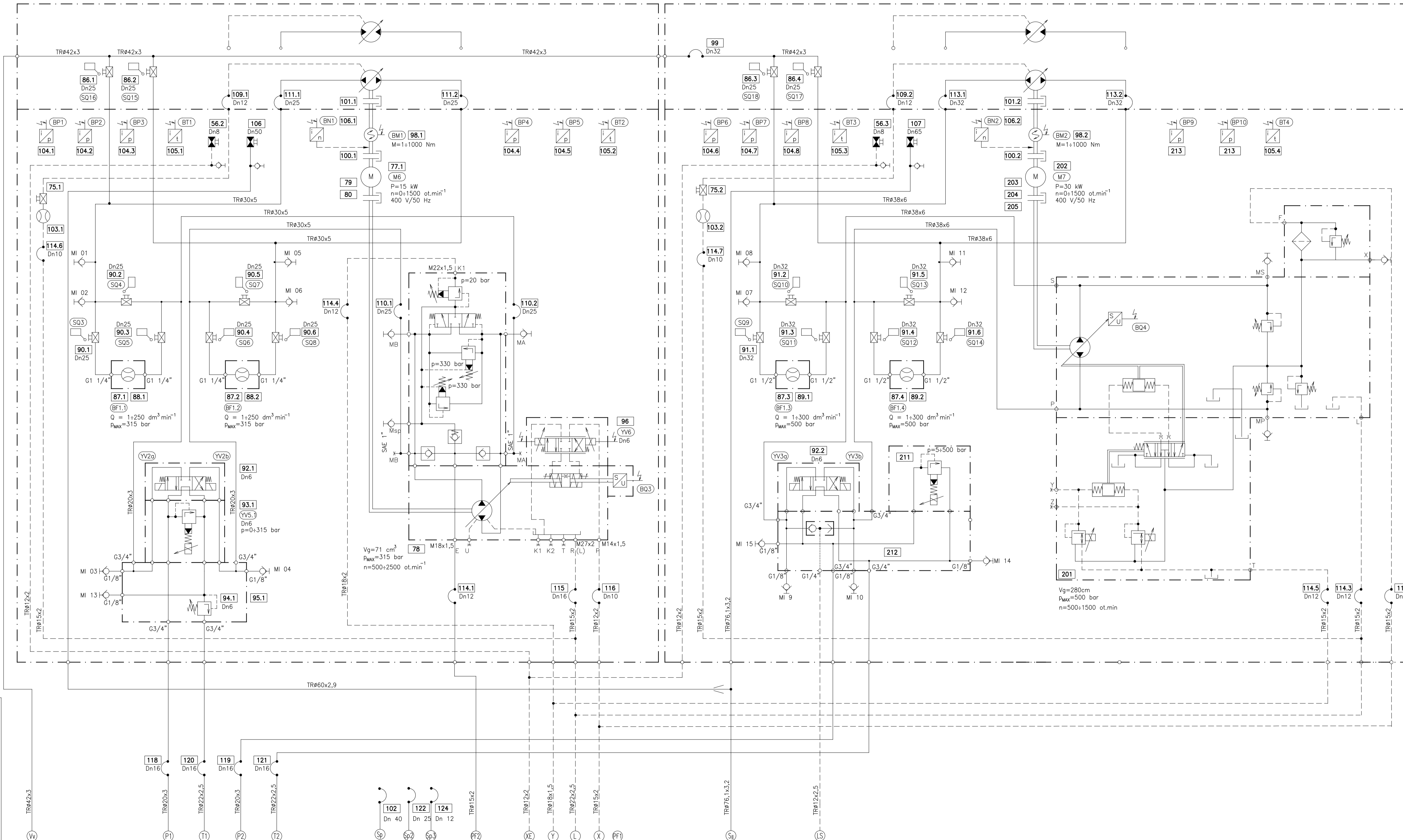
ZKUŠEBNÍ STEND HG A HM PRO V_g < 280 \text{ ccm}
