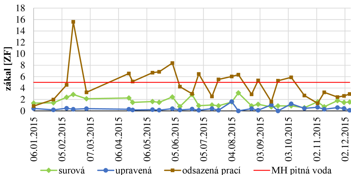
Graf 5.1 Naměřené hodnoty zákaly v průběhu roku 2015
