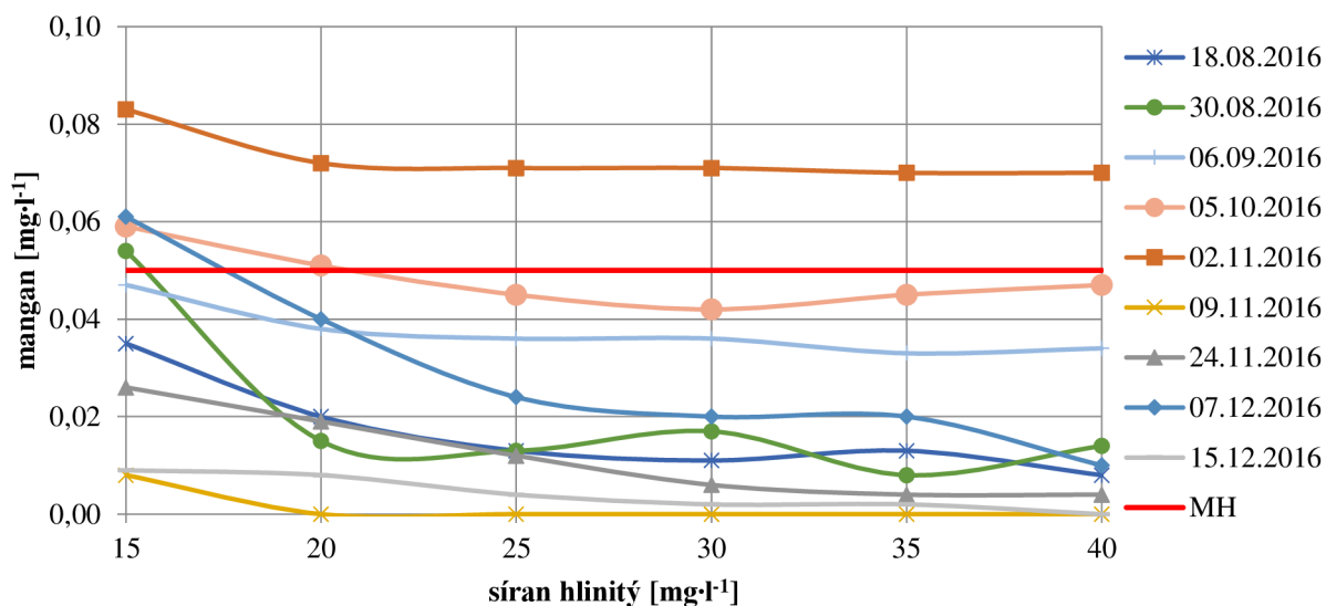
Graf 6.17 Koncentrace manganu po provedení koagulačních zkoušek
