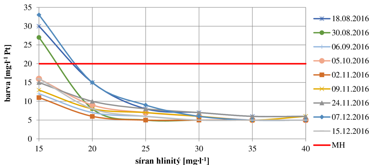
Graf 6.13 Hodnoty barvy po provedení koagulačních zkoušek
