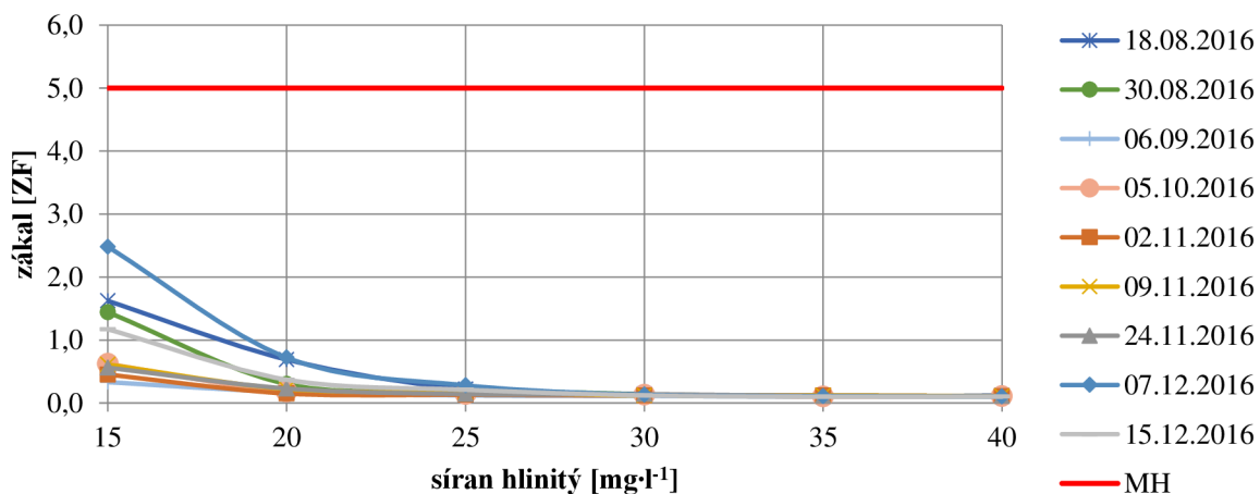
Graf 6.12 Hodnoty zákaly po provedení koagulačních zkoušek
