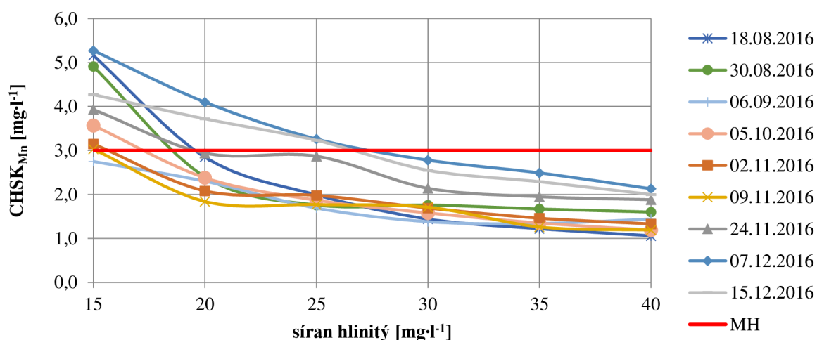
Graf 6.14 Hodnoty chemické spotřeby kyslíku po provedení koagulačních zkoušek
