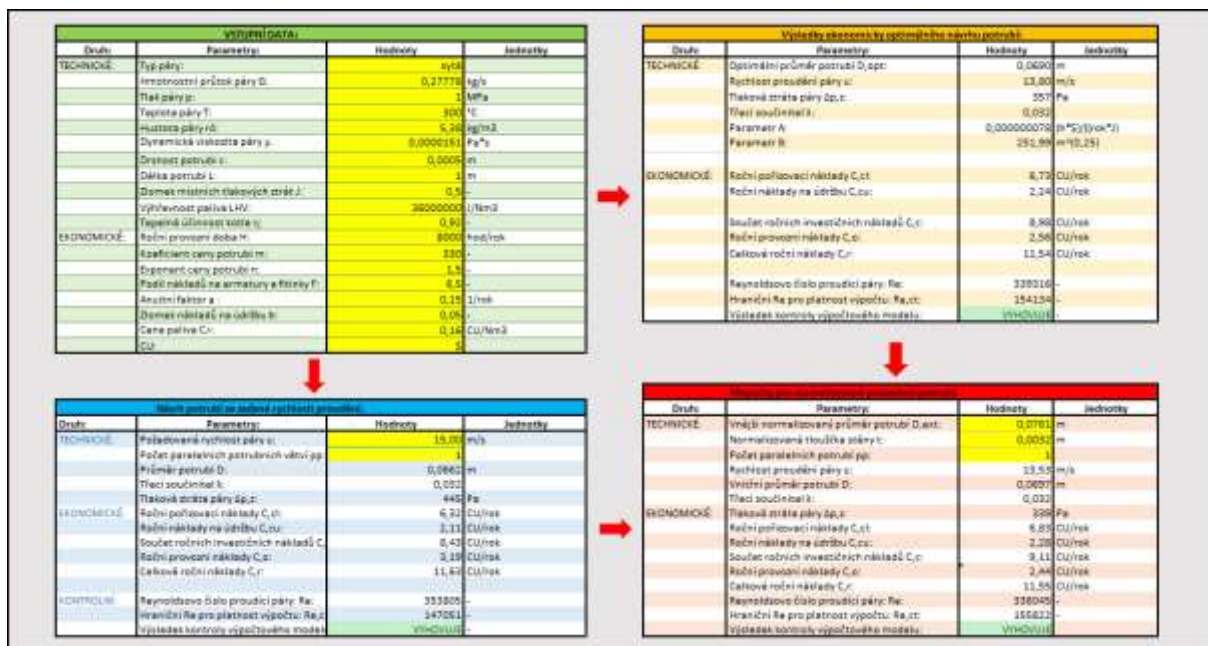
Obr. 2 Výpočetní nástroj pro výpočet ekonomicky optimálního průměru potrubí
