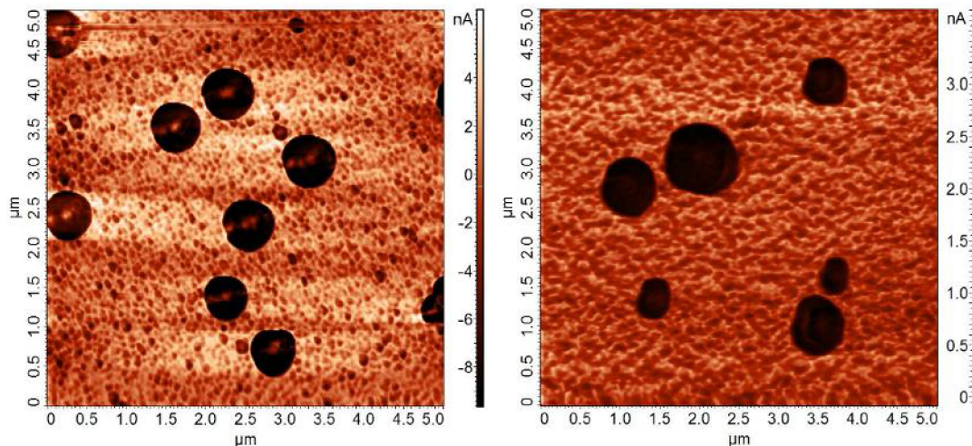
Obr. 53: Vľavo AFAM snímka pp-TVS vrstvy (50 W), vpravo AFAM snímka vrstvy Si.
