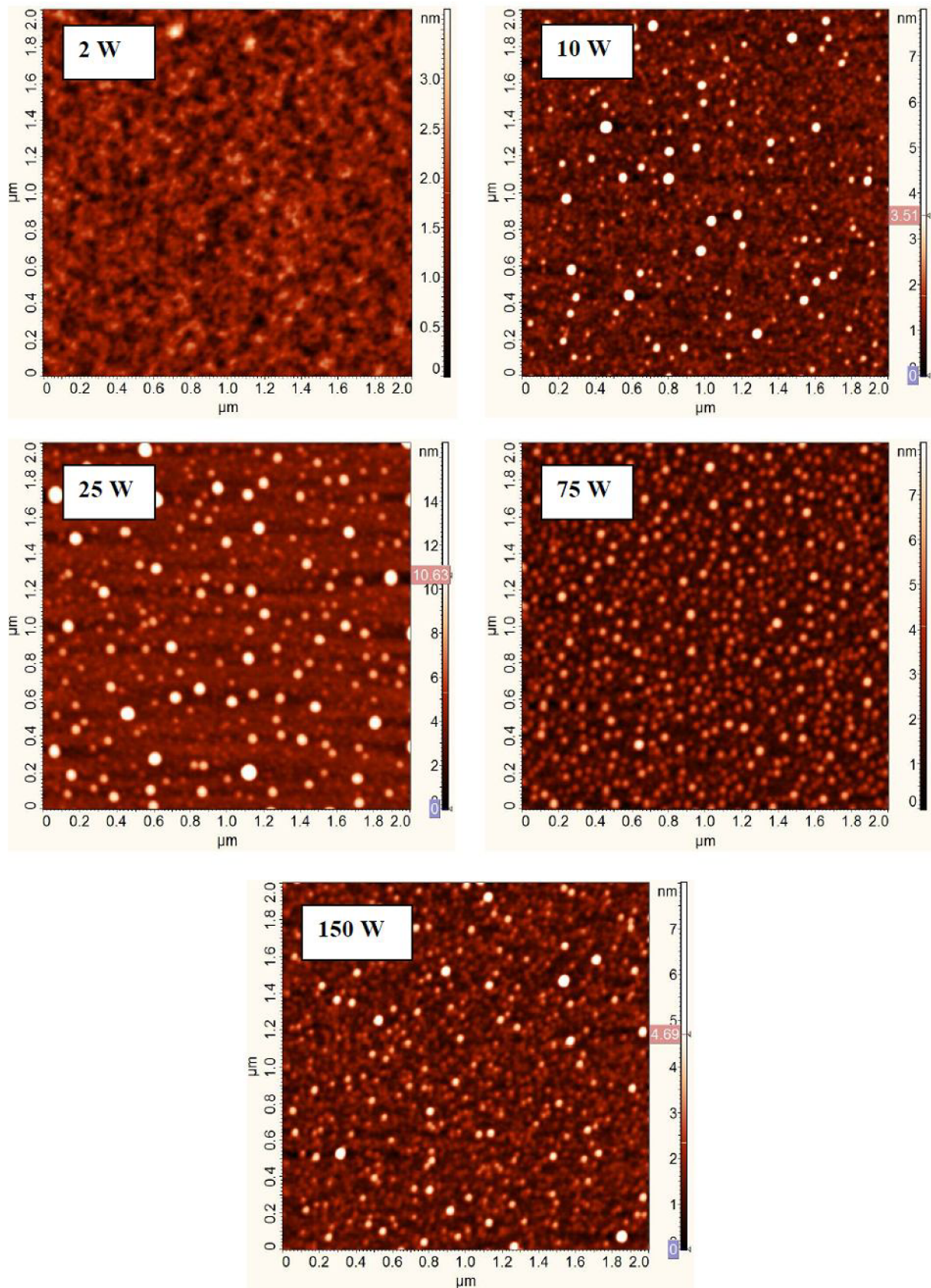
Obr. 75: Výškové mapy o ploche 2 x 2 \mu\text{m} vrstiev pripravených zo zmesi TVS a kyslíku (3,5 sccm).
