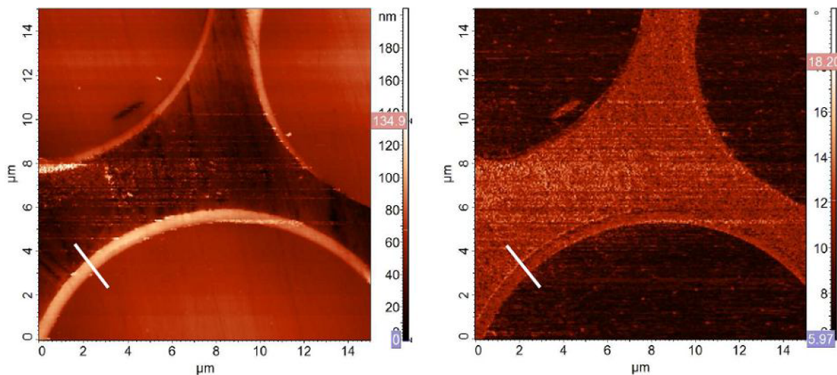
Obr. 87: Vľavo je topografia plochy 15 \times 15 \mu\text{m} ukazujúca vlákna upravené polymérou vrstvou umiestnené v matrici, vpravo je odpovedajúca mapa fázového kontrastu.
