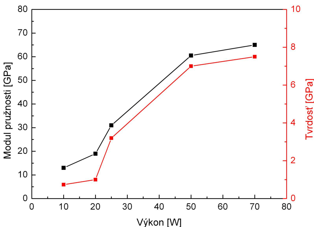
Obr. 52: Závislosť modulu pružnosti a tvrdosti na výkone použitého výboja pre vrstvy pripravené v kontinuálnom režime.
