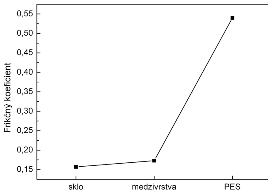
Obr. 91: Frikčný koeficient jednotlivých fází kompozitu.
