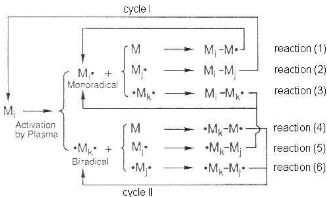
Obr. 4: Zovšeobecný mechanizmus plazmovej polymerácie [11].
