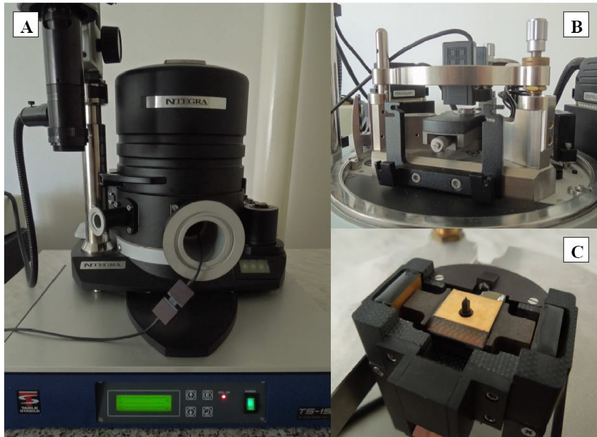
Obr. 39: A – Celkový pohľad na systém NTEGRA pri vykonávaní nanomechanických skúšok, B – Záber na hlavu TriboScope umiestnenú nad vzorkou na stolčeku, C – Detail na prevodník hlavy TriboScope (v strede je testovací hrot).
