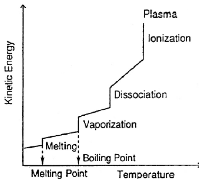
Obr. 1: Energetická závislosť skupenských stavov [1].
