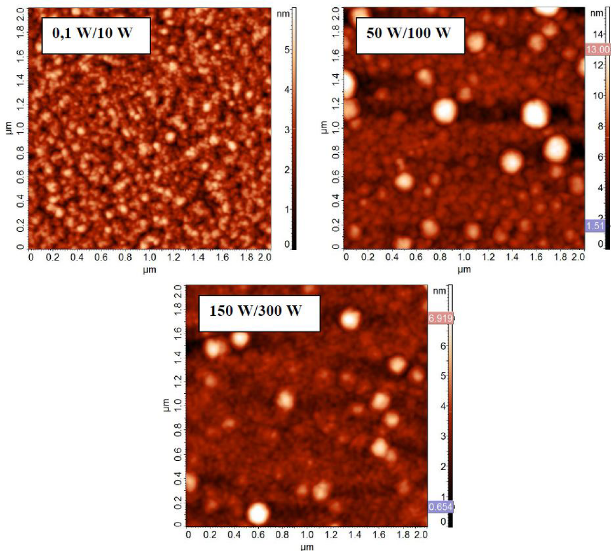
Obr. 61: Ukážka topografie vrstiev pripepravených pri rozličných efektívnych (a hrubých) výkonoch.
