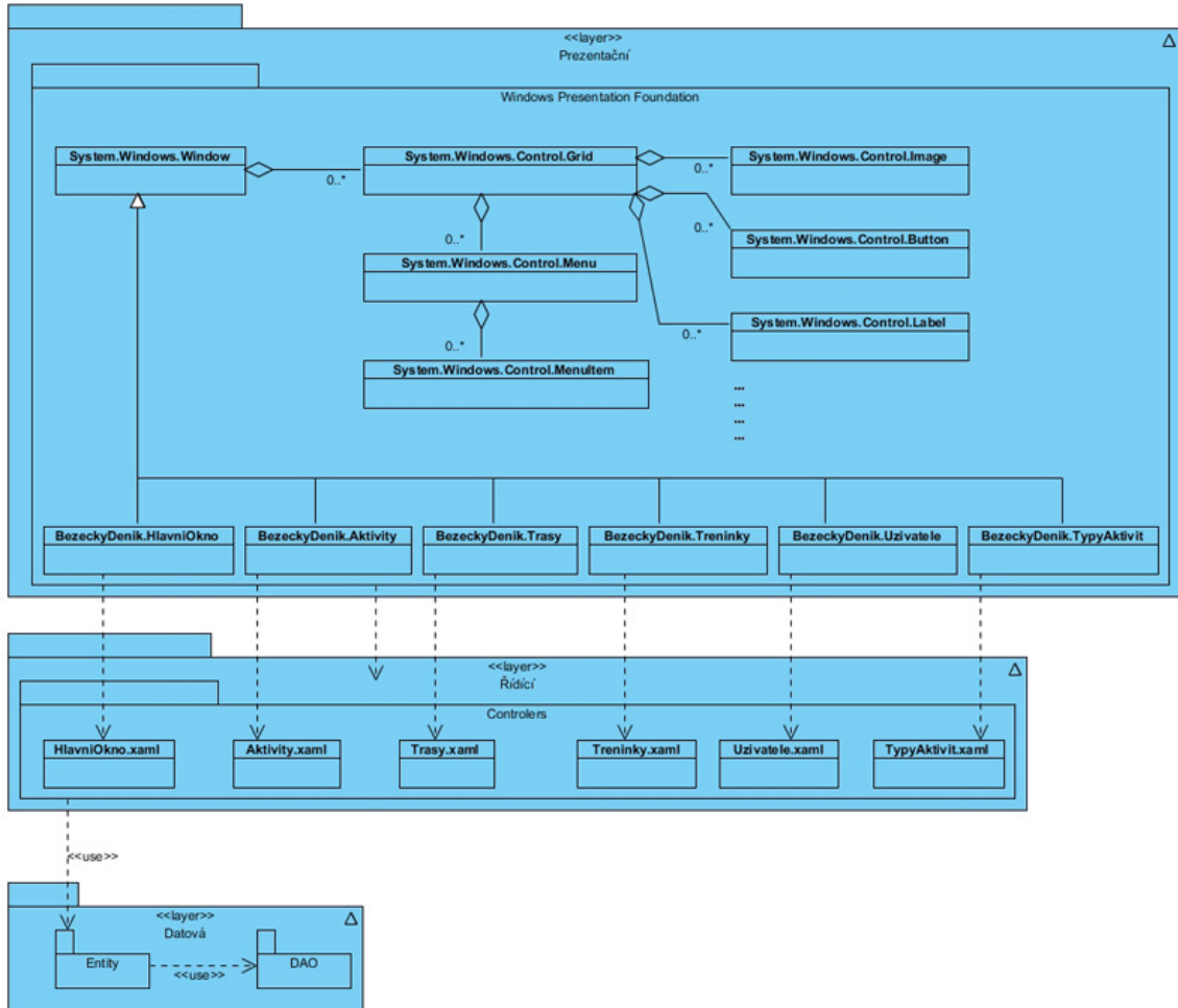
Obrázek 4.6: Rozdělení aplikace.
