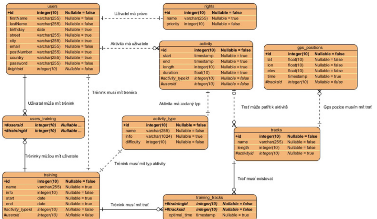
Obrázek 4.5: ER diagram.
