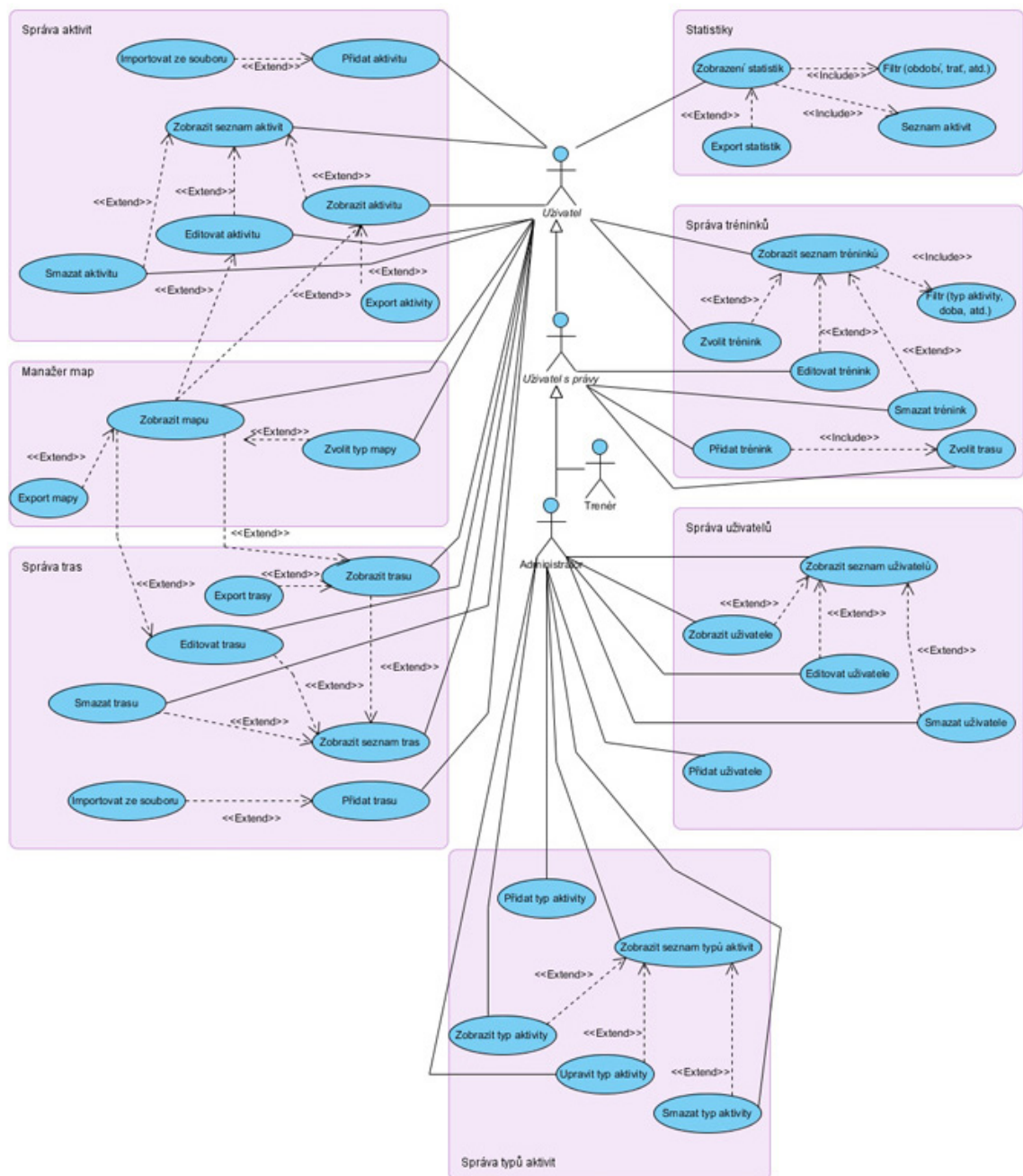
Obrázek 4.1: Případy užití.
