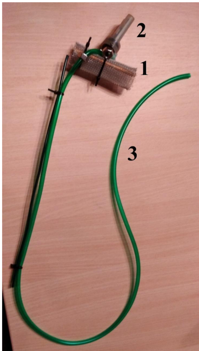
Obrázek 12: Bioindikační sondice. 1 - nerezová síť vyložená uhelovou síťovinou, 2 - kontinuální teploměr HOBO WARE, 3 - hadička sloužící k odběru hyporeální vody. Foto: Marta Rojtová, 2021.
