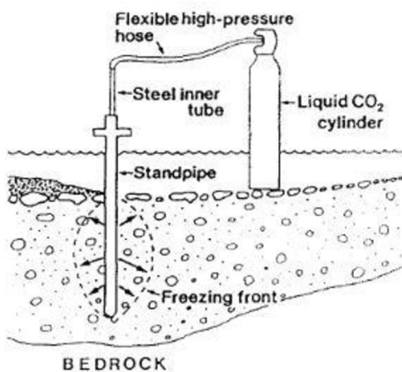
Obrázek 35: Vizualizace metodiky odebrání vzorků říčního dna zmrazováním. Převzato z Thoms (1992).
