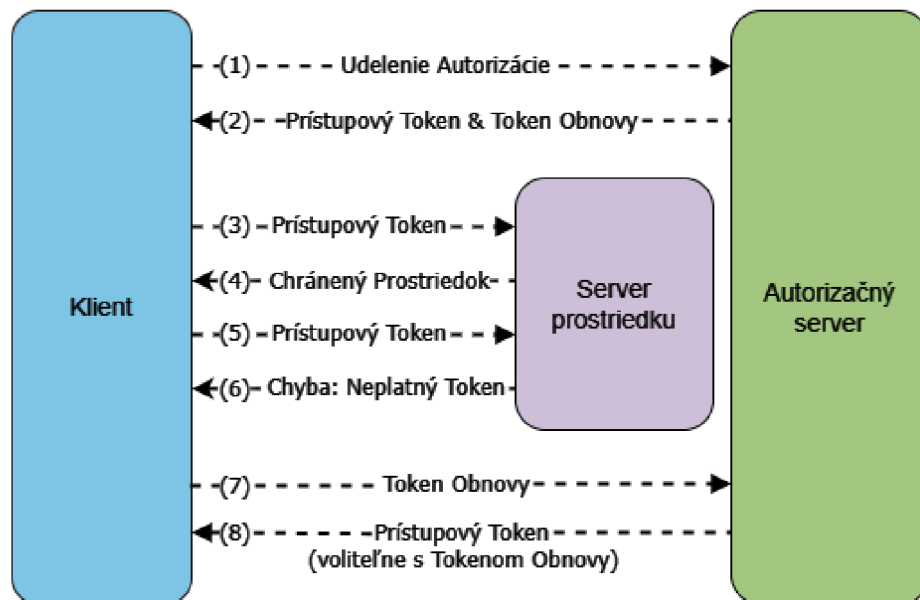
Obr. 4.3: Obnovenie expirovaného prístupového tokenu, prebratý z [23]
