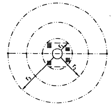
KONZOLA L ZDOVJENÁ, 2 PODPĚRY, 2 VZPĚRY NA BETONOVÝ STOŽÁR JB
