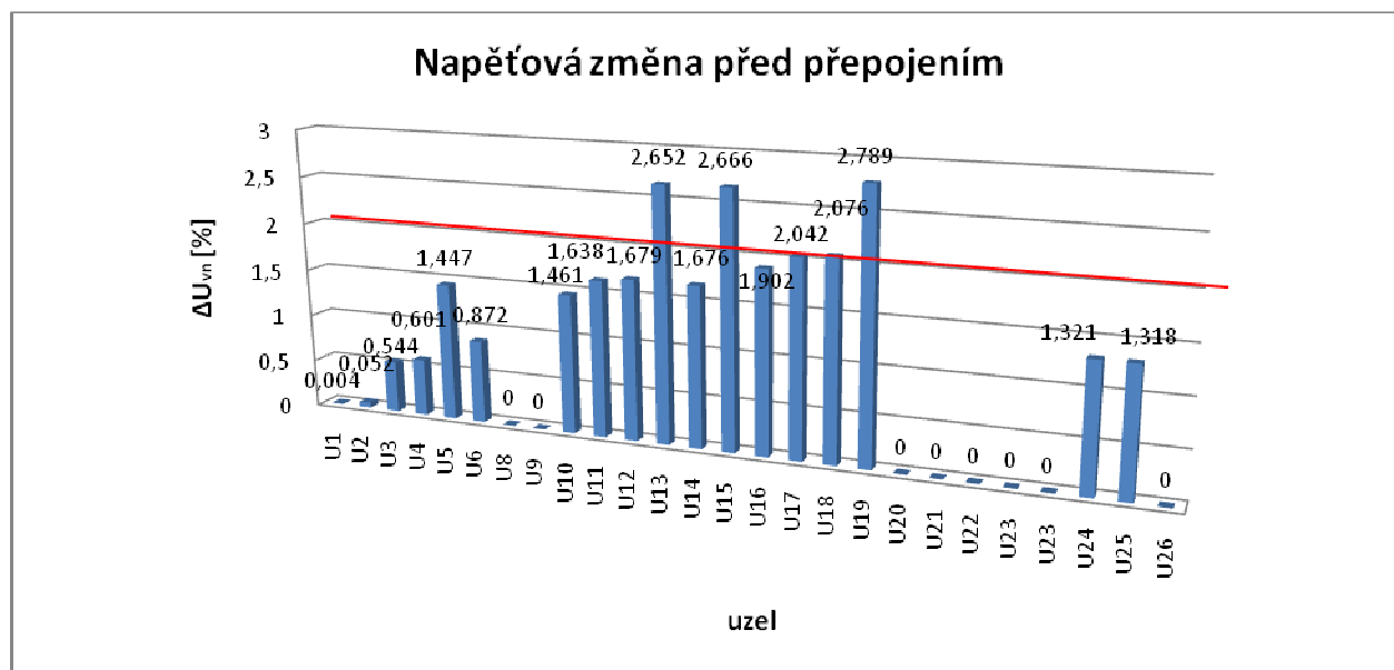
Obrázek 4-3 Napěťové změny linky VN 350 před přepojením
