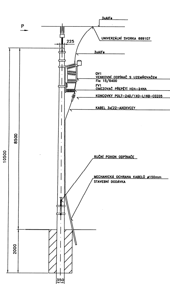
KONZOLA L ZDOVJENÁ, 2 PODPĚRY, 2 VZPĚRY NA BETONOVÝ STOŽÁR JB
