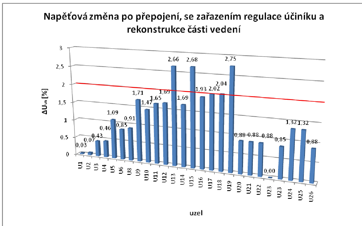
Obrázek 4-8 Napěťová změna na lince VN 350 po přepojení, se zařazením regulace účiníku a rekonstrukce části vedení
