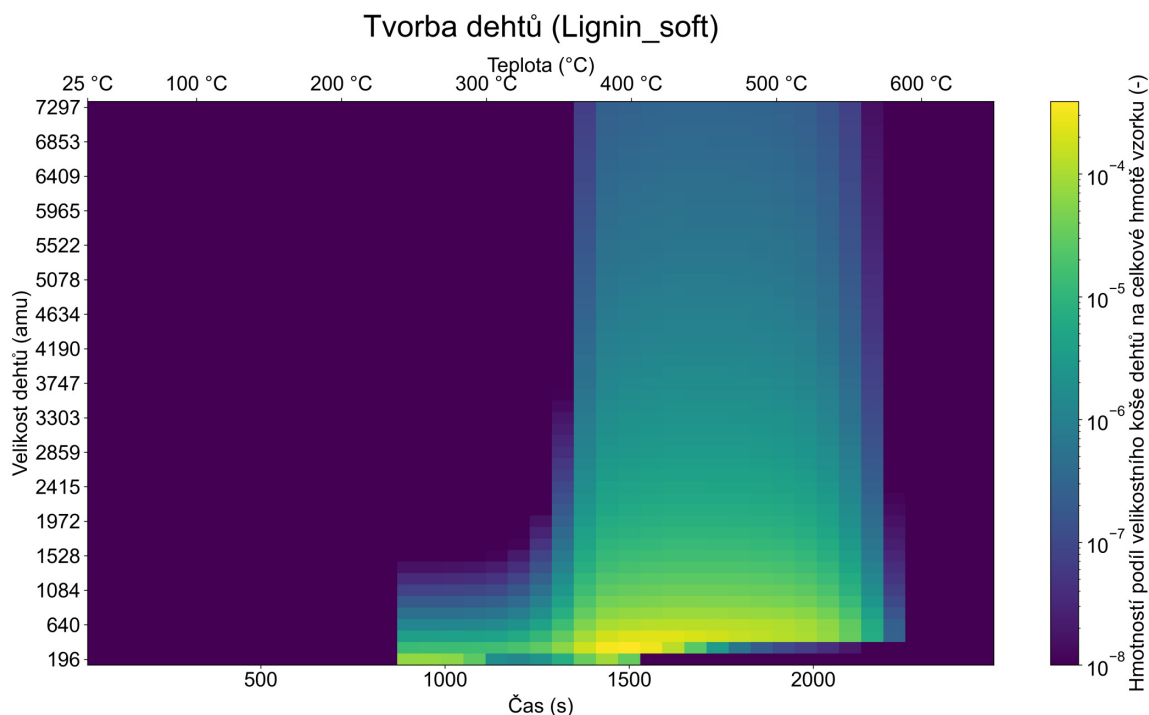
Obrázek 5.10: Tvorba dehtů v modelu Bio-CPD pro pyrolýzu ligninu pro měkké dřevo. Žlutá barva vyjadřuje vysoký hmotnostní podíl dehtů v daném čase a velikostním koši, modro-fialová barva pak vyjadřuje nízkou nebo žádnou tvorbu dehtů.
