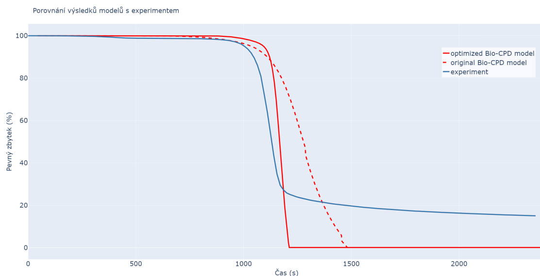
Obrázek 6.13: Porovnání úbytku hmotnosti experimentálního vzorku celulózy (modrá plná čára) a modelu Bio-CPD s původními kinetickými parametry (přerušovaná červená čára) a s nulovým parametrem odchylky \sigma_b (plná červená čára).
