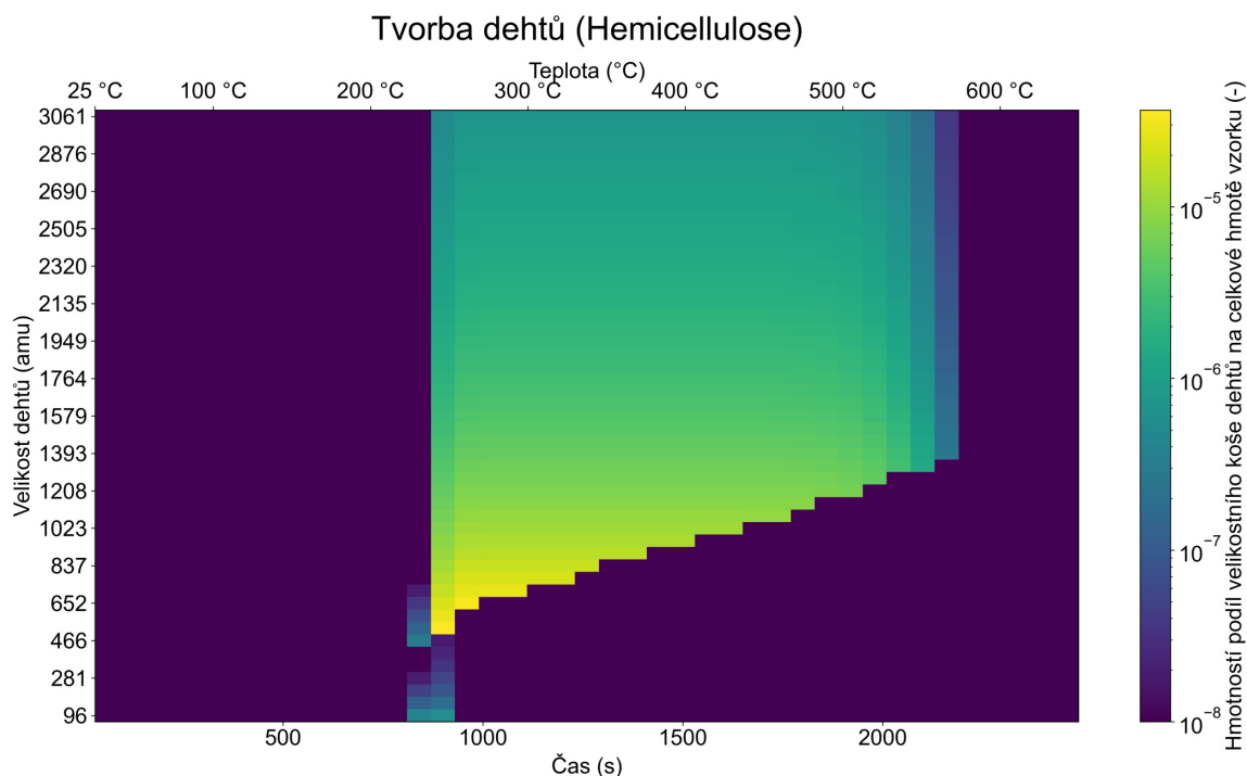
Obrázek 5.4: Tvorba dehtů v modelu Bio-CPD pro pyrolýzu hemicelulózy. Žlutá barva vyjadřuje vysoký hmotnostní podíl dehtů v daném čase a velikostním koši, modro-fialová barva pak vyjadřuje nízkou nebo žádnou tvorbu dehtů.
