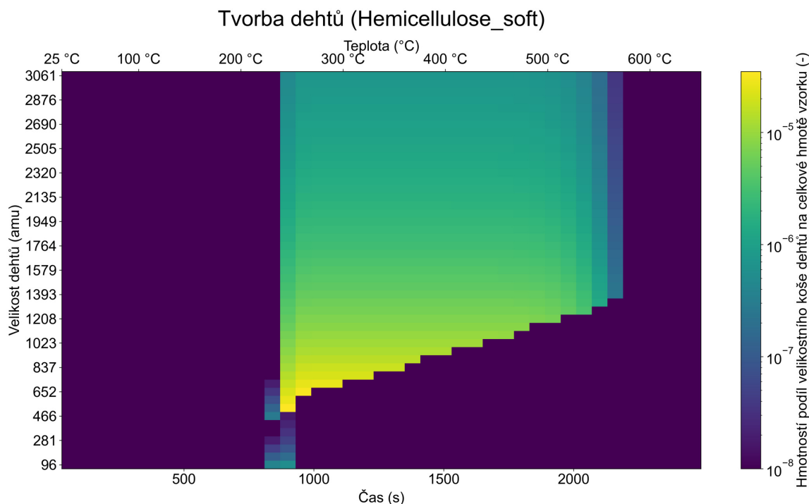
Obrázek 5.6: Tvorba dehtů v modelu Bio-CPD pro pyrolýzu hemicelulózy pro měkké dřevo. Žlutá barva vyjadřuje vysoký hmotnostní podíl dehtů v daném čase a velikostním koši, modro-fialová barva pak vyjadřuje nízkou nebo žádnou tvorbu dehtů.
