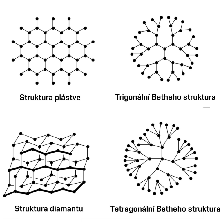
Obrázek 4.1: Repräsentace reálných struktur (včelí plástev a diamant) a Betheho pseudostruktur pro koordinační číslo 3 a 4 [22].
