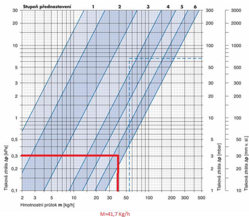
Obrázek 2.8.3 Regulace nejuzdálenějšího tělesa S3 [15]
