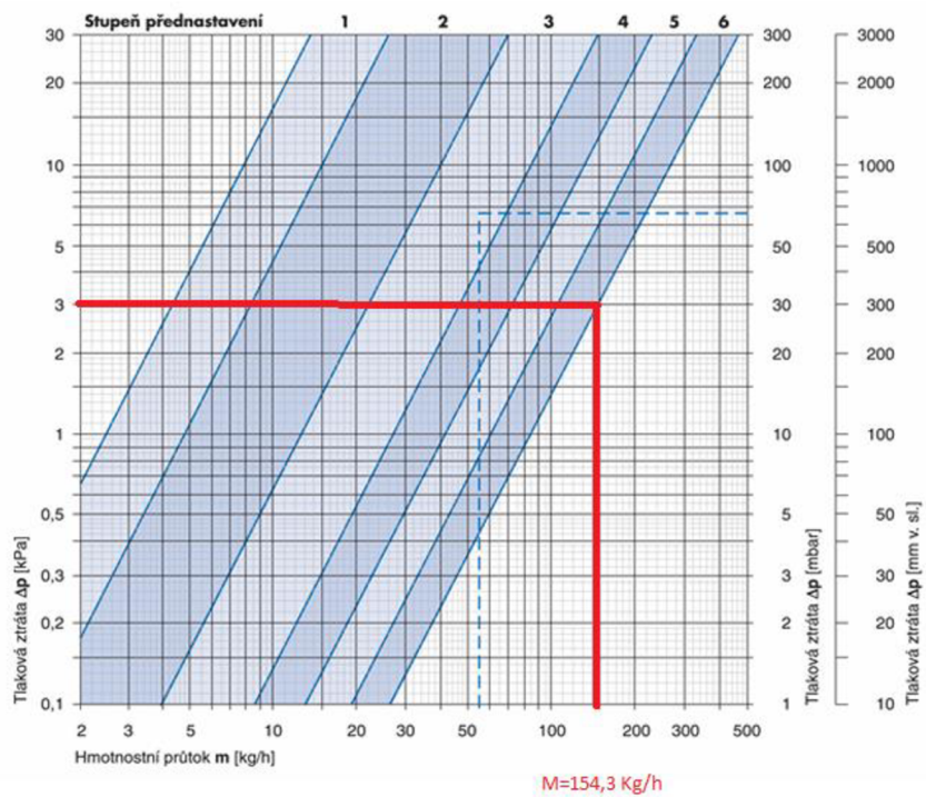
Obrázek 2.8.2 Regulace nejbzdálenějšího tělesa S2 [15]
