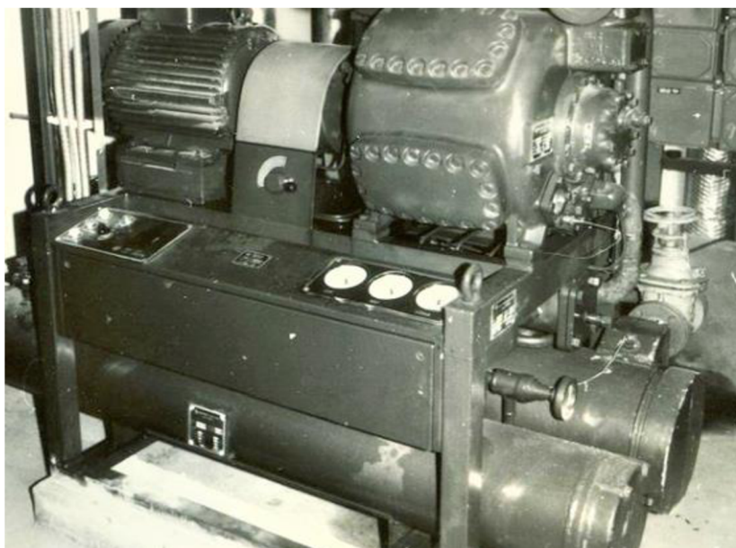
Obrázek 1.2 Historické tepelné čerpadlo z ČDK Choceň nainstalované v r. 1982 [1]
