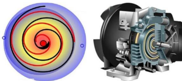
Obrázek 1.5.1.1 Scroll kompresor [5]
