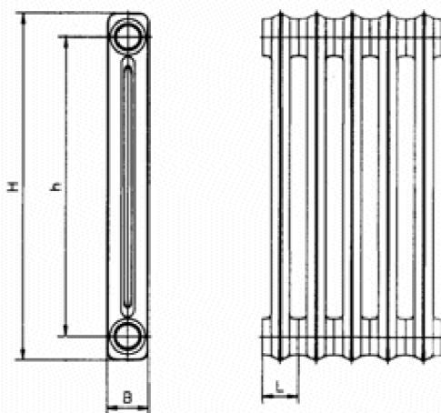
Obrázek 1.6.2 Článkové otopné těleso [10]
