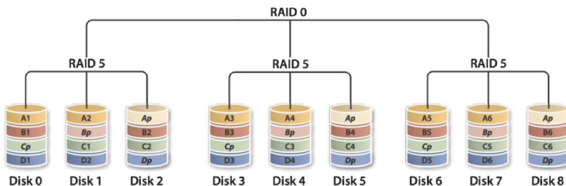
Obrázek 7 RAID 50
