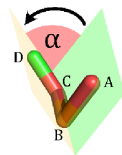
Obrázek 10 Ukázka měření dihedrálního úhlu
