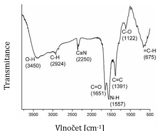
Obrázek 5 Spektrum CD získané pomocí FTIR (převzato a upraveno z 52)
