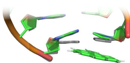
Obrázek 13 Porovnání výchozí vzájemné polohy terminálních bází a změny parametru buckle vyvolán nasednutím CD_pure
