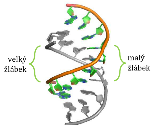
Obrázek 3 Velký a malý žlábek duplexu RNA
