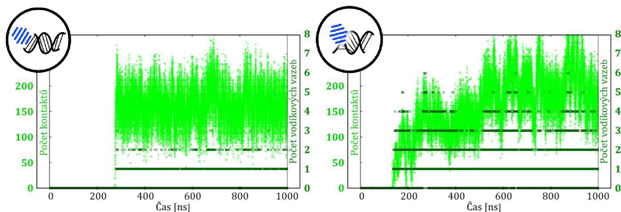
Obrázek 17 Grafy počtu kontaktů a vodíkových vazeb pro modely AU_CD_NH3_3 (vlevo) a AU_CD_NH3_5 (vpravo)
