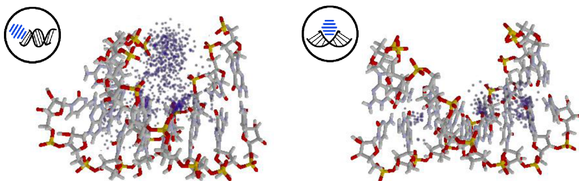
Obrázek 27 Porovnání hustotní mapy draselných iontů ve velkém žlábku CG_CD_NH3_3 (PI na terminální báze duplexu) a CG_CD_NH3_4 (HB s páteří duplexu)
