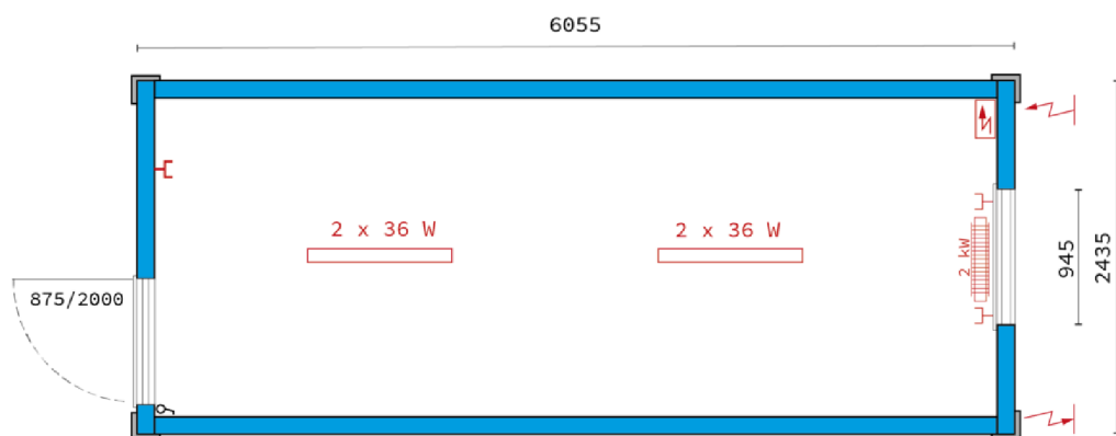
Obr. 19 Pôdorys stavebného kontajner ToiToi KK1 [5]
