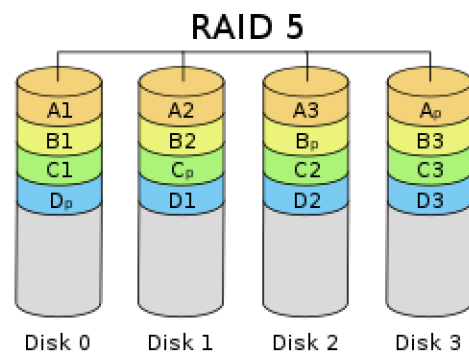
Obrázek 12: RAID 5
