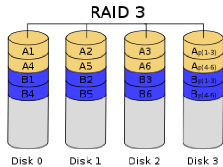
Obrázek 11: RAID 3
