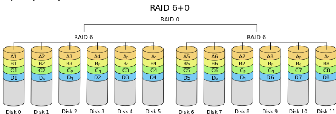
Obrázek 20: RAID 6+0
