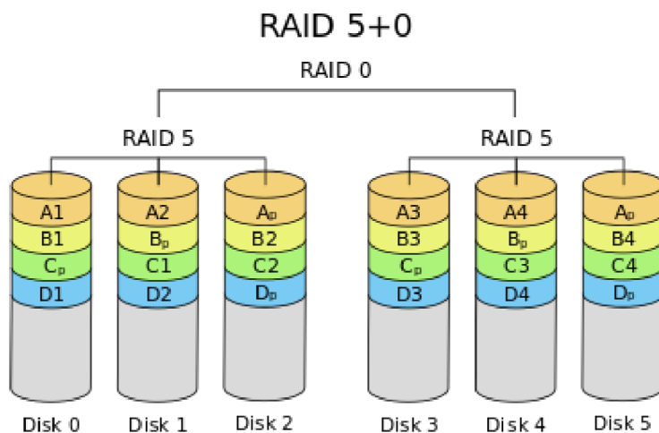
Obrázek 18: RAID 5+0
