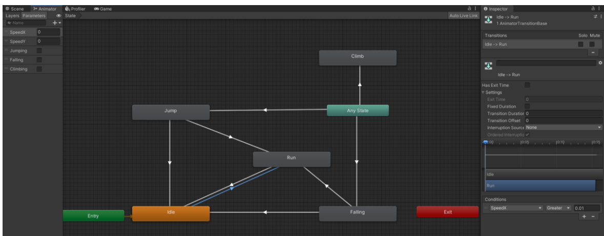
Obrázek 19: Stavy animací v okně „Animator“ (vlastní zpracování)
