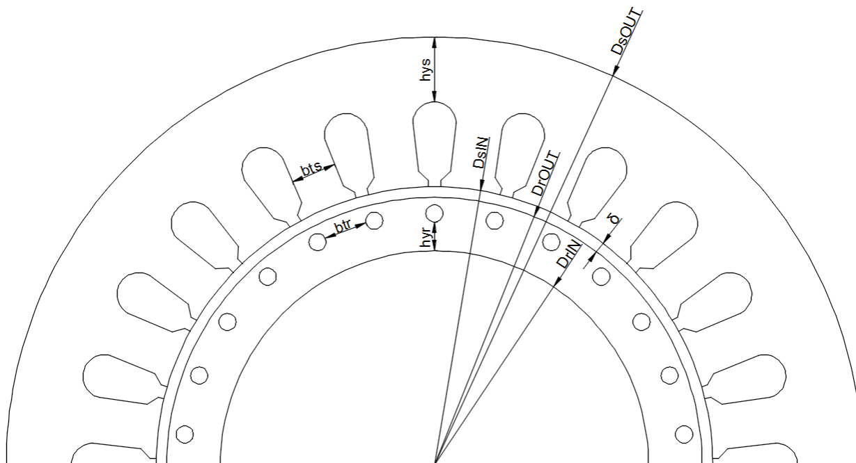
Obrázek 3-1 Hlavní rozměry stroje
