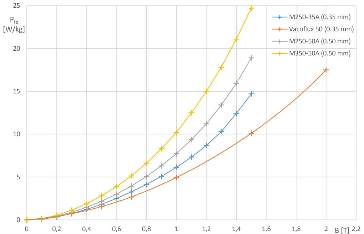
Obrázek 2-3 Srovnání měrných ztrát různých elektrotechnických plechů při f=200 Hz. Převzato z [3][9]
