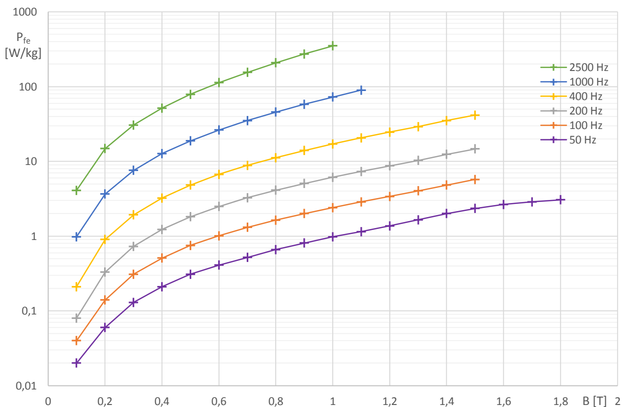
Obrázek 2-2 Ztrátové křivky plechu M250-35A – závislost P_{fe}=f(B) . Převzato z [3]
