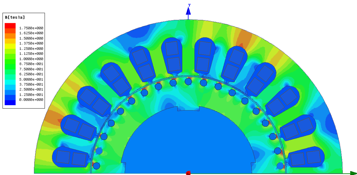
Obrázek 4-9 Rozložení magnetického pole při jmenovitých otáčkách stroje s uzavřenými rotorovými drážkami
