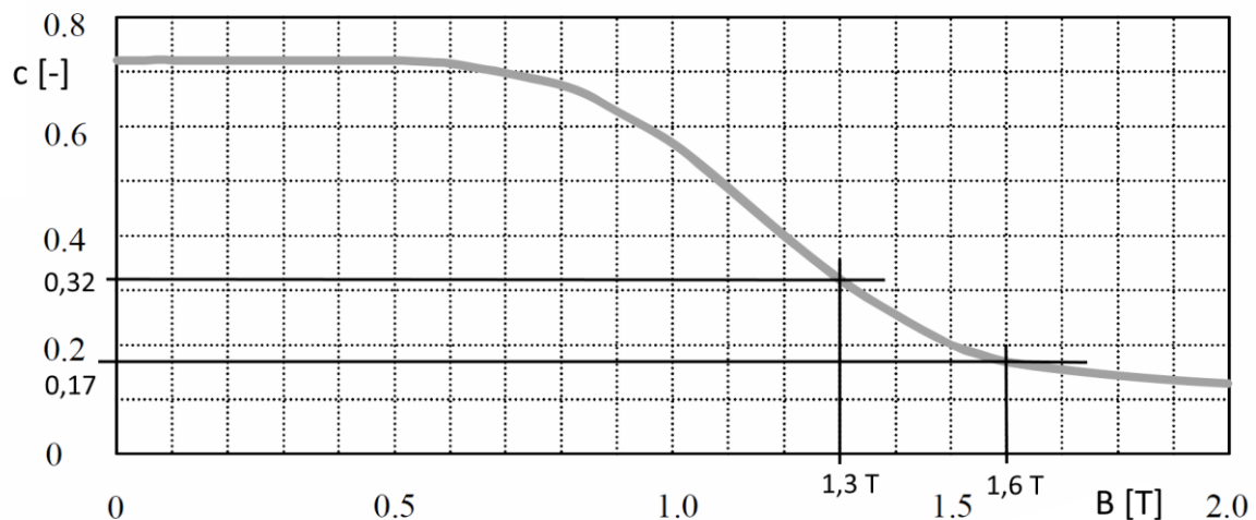
Obrázek 3-7 Závislost koeficientu c na magnetické indukci ve jhu statoru a rotoru pro výpočet magnetického napětí. Převzato z [1]
