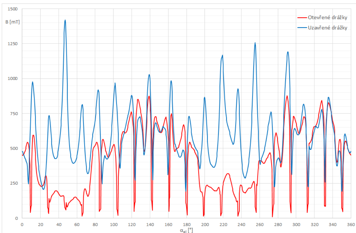
Obrázek 4-5 Průběh magnetické indukce nad rotorovými tyčemi při simulaci naprázdno
