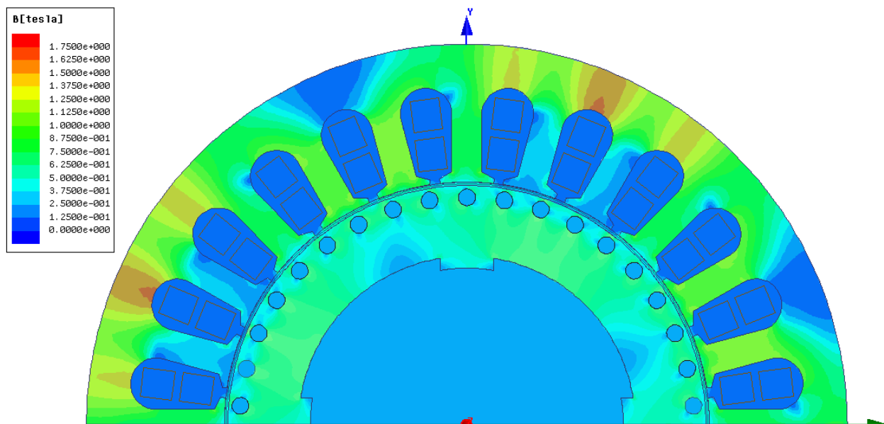
Obrázek 4-4 Rozložení magnetického pole ve stavu naprázdno
