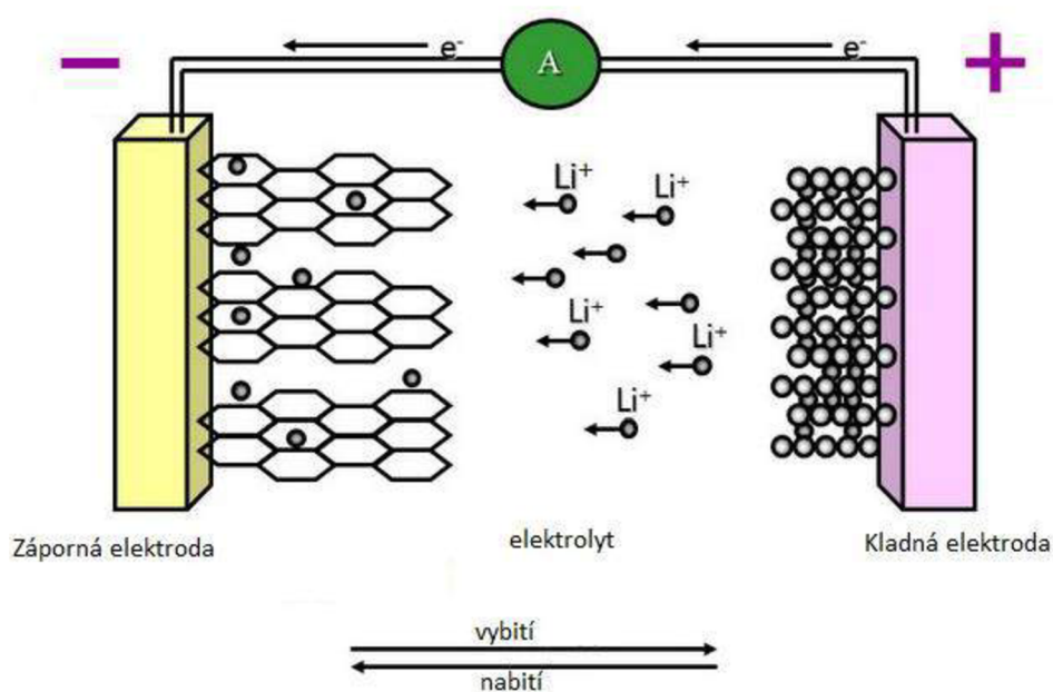
Obr. 4 Princip Li-Ion článku [12]
