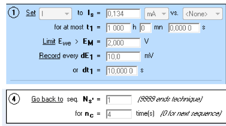
Obr. 27 Nastavení nabíjecího proudu a počtu cyklů u GCPL v programu EC-lab
