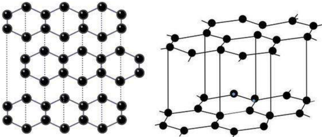
Obr. 8 Struktura grafitu [20] [21]
