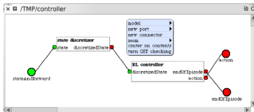
Obrázek 3.3: Inspektor sdružených modelů
