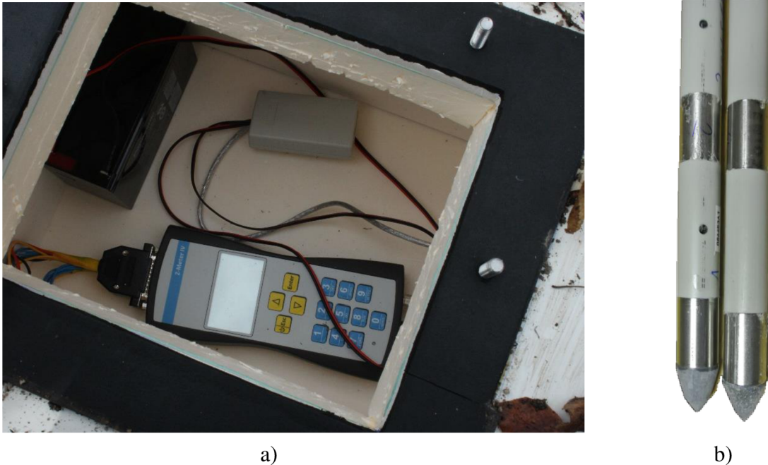
Obr. 2-14: Temperovaný úložný box s přístrojem, kabeláží, záložní Pb baterií a jednotkou USB a), detail měřících trubic s elektrodami EIS s teploměry b)
