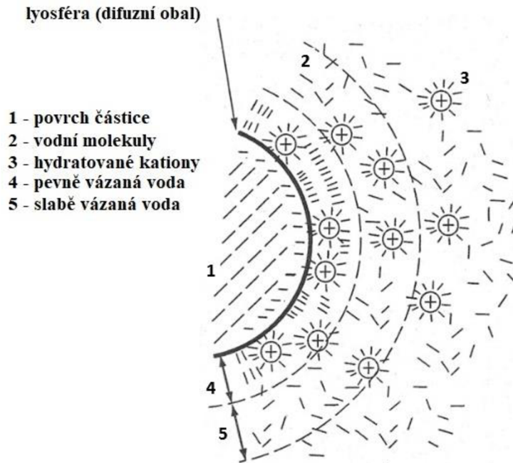
Obr. 2-3: Difuzní obal minerálních povrchů [6]
