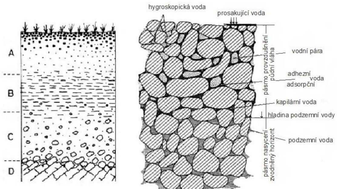
Obr. 2-5: Schéma vertikálního řezu zeminou [16] (vlevo) s návazností rozdělení podzemní vody (vpravo)
