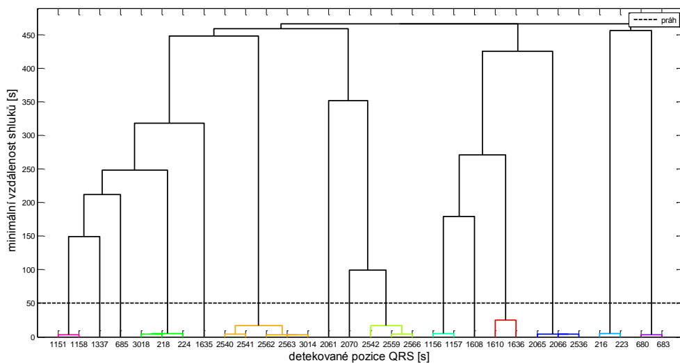
Obr. 4.2: Shluková analýza s prahováním.
