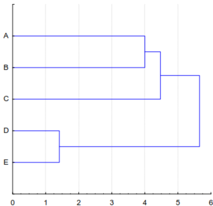
Obr. 3.6: Výsledný dendrogram (21)
