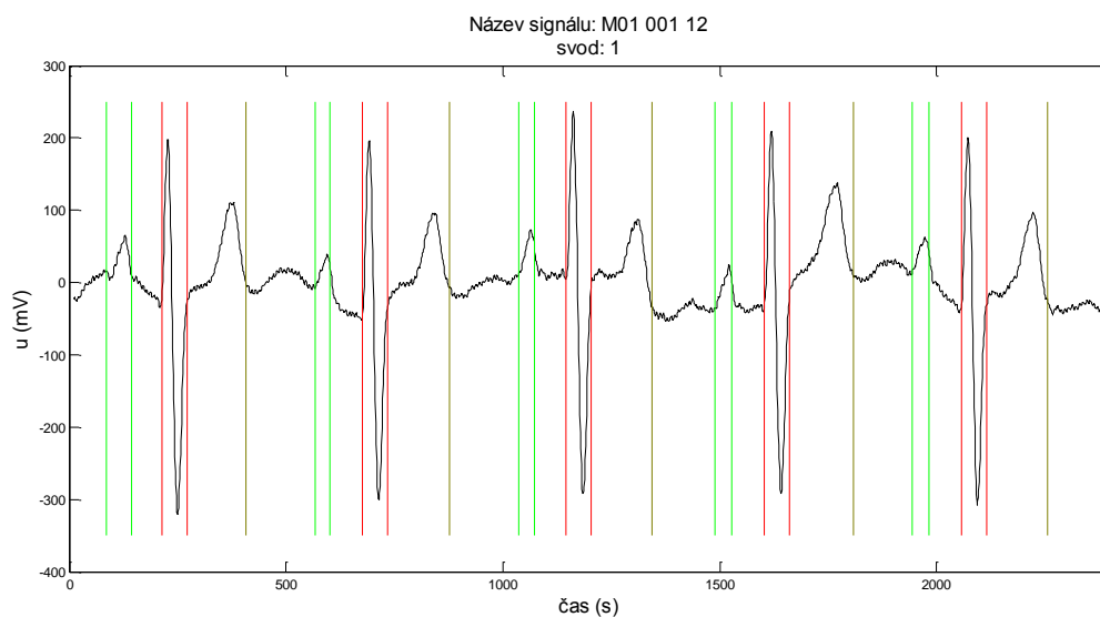
Obr. 4.17: Detail výsledku rozměření signálu z obr. 4.12
