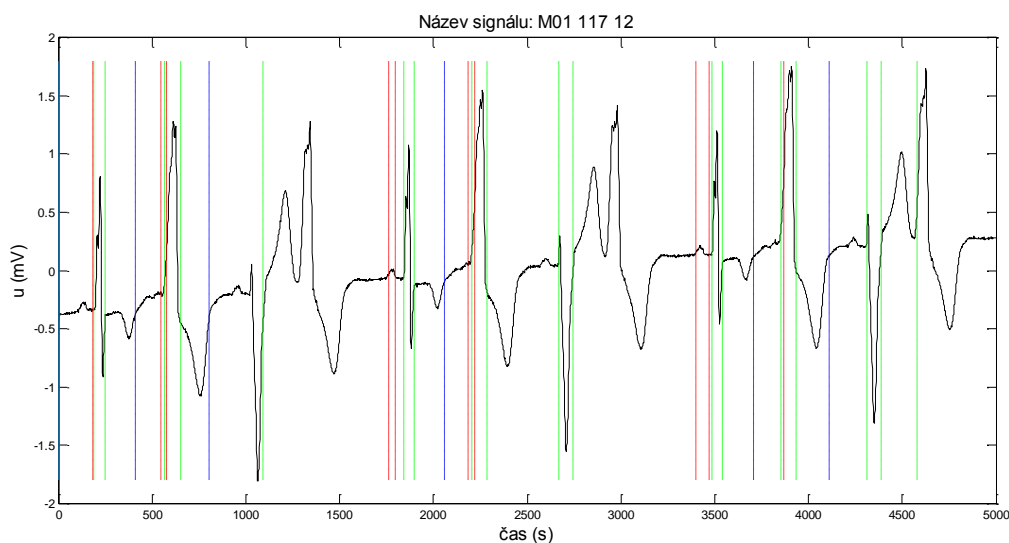
Obr. 4.27: Výsledek rozměření signálu M01 001 12. Kombinace metod.
