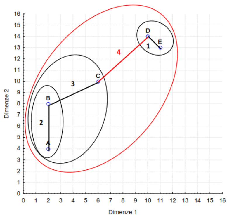
Obr. 3.5: Vytvořené shluky při použití výpočtu euklidovské matice a metody nejbližších sousedů. (21)
