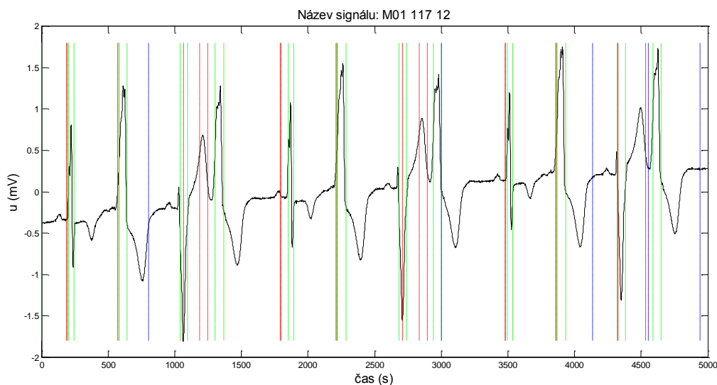
Obr. 4.26: Výsledek rozměření signálu M01 117 12. Metoda založena využívající kvantizačního prahu.
