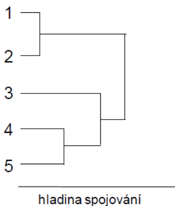
Obr. 3.3: Ukázka dendrogramu (2)
