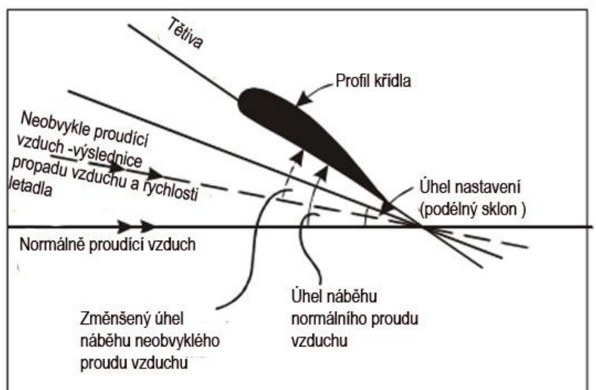
Obr 4.4 Výslednice směru nabíhajícího vzduchu [10].
