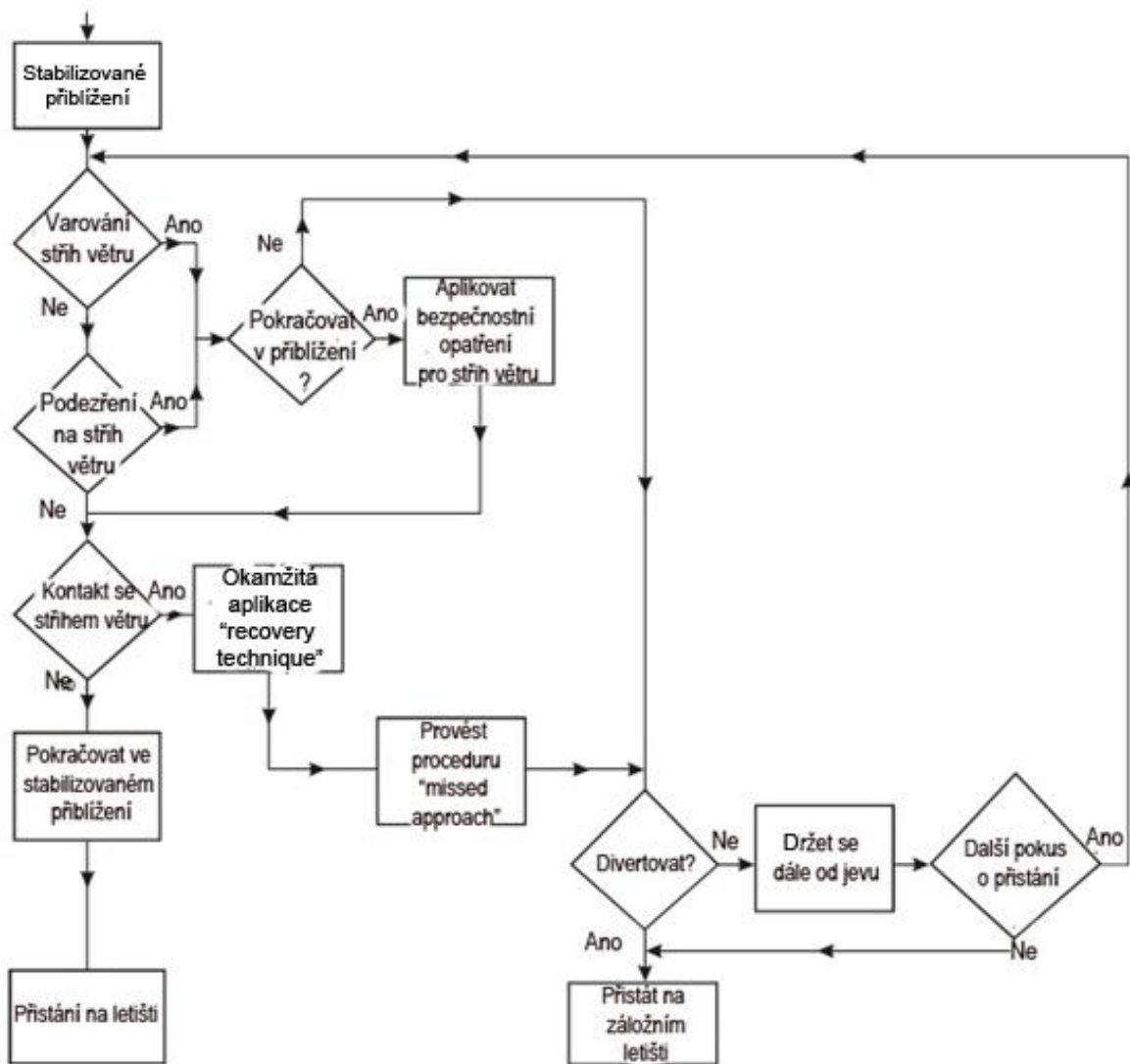
Obr. 4.6 Postup řešení střetu se stříhem větru [10].
