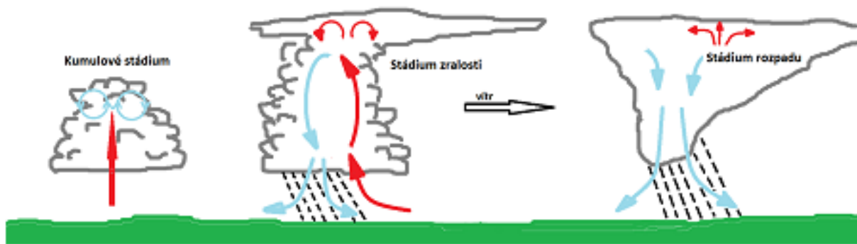
Obr. 3.8 Stádia bouřky [27].
