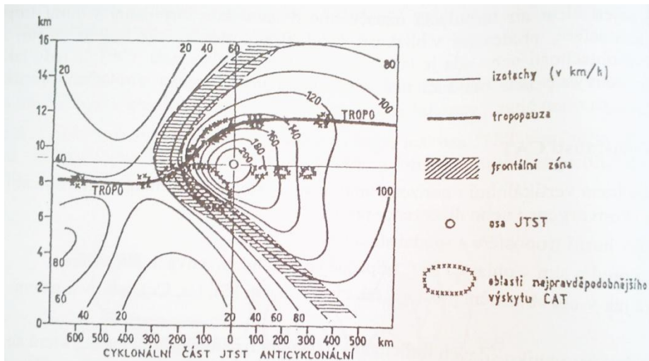
Obr. 3.15 Řez JTST s výskytem turbulence [12].
