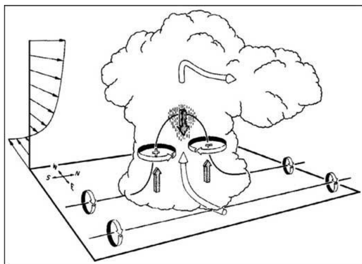
Obr. 3.13 Vznik supercely [73].
