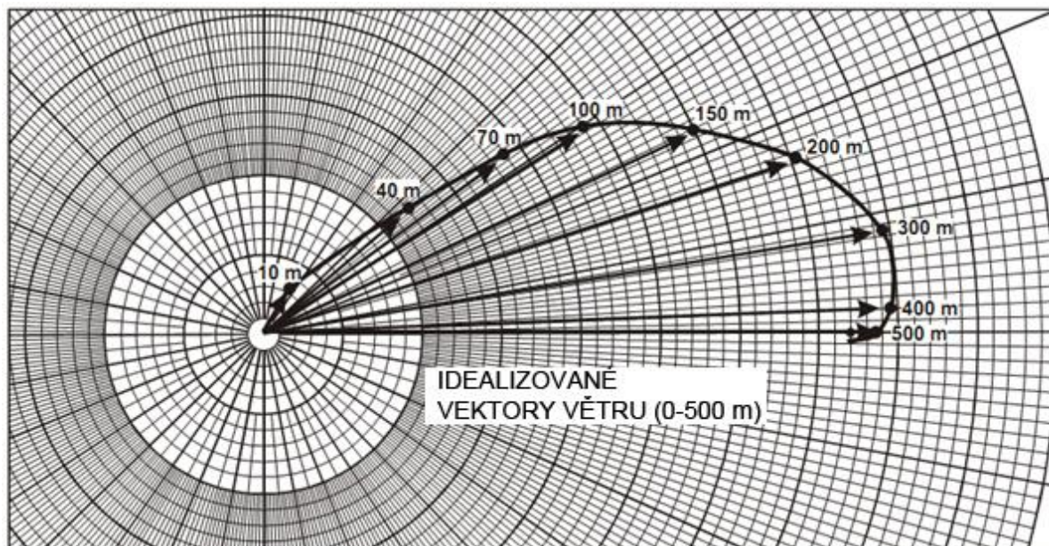
Obr. 3. 3 Ekmanova spirála [10].
