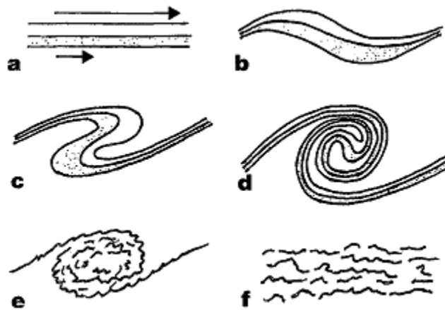
Obr. 3.14 Vznik turbulence z Kelvin a Helmholtzovy vlny [23].
