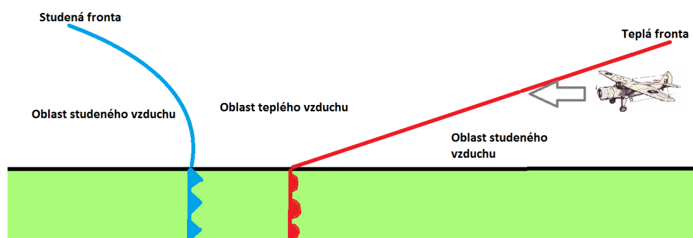
Obr. 3. 7 Fronty [autor].
