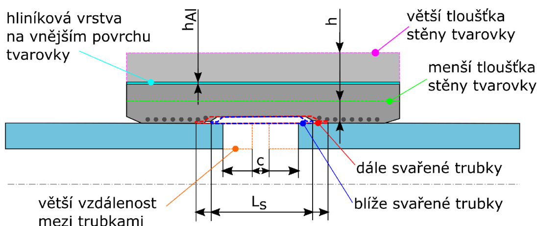
Obr. 4.2: Schematické znázornění uvažovaných modifikací
