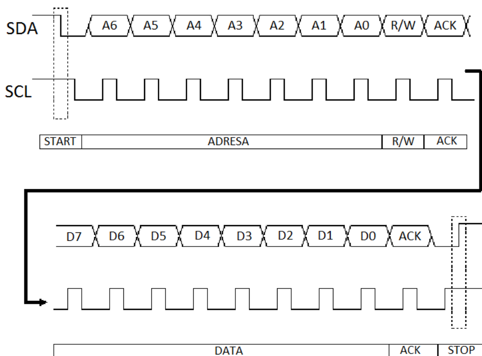
Obr. 7 Průběh komunikace na sběrnice I2C
