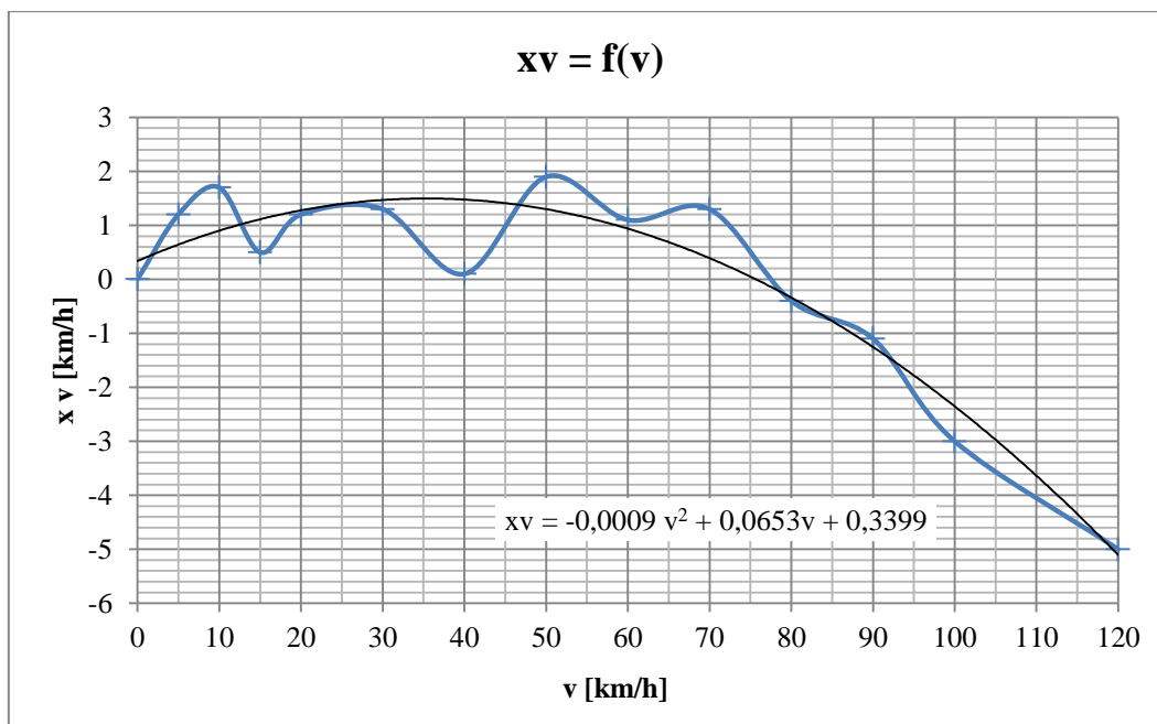
Obř. 21 Kalibrační funkce rychlosti větru
