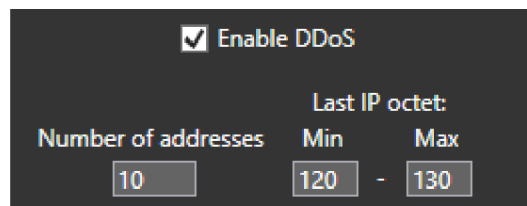
Obr. 5.8: Nastavenia DDoS
