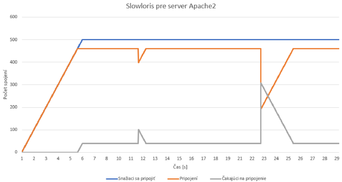
Obr. 6.1: Graf priebehu útoku Slowloris
