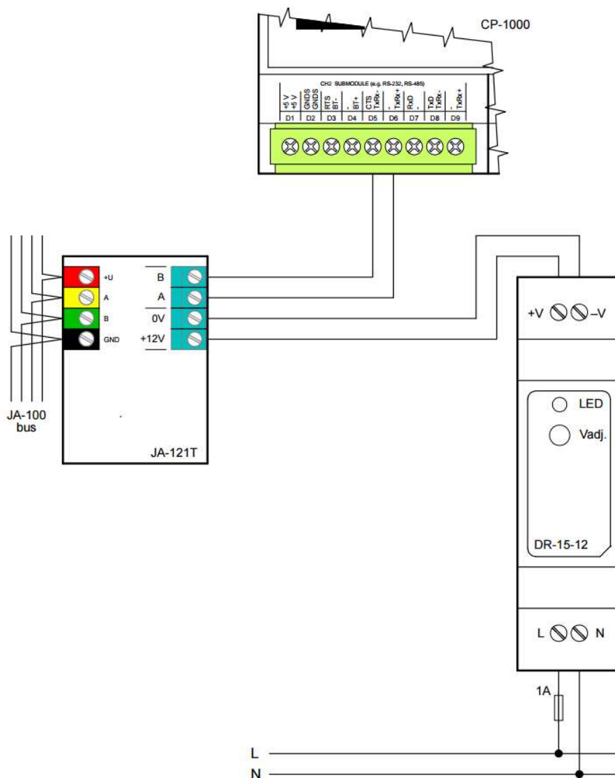
Obr. 4-2: Připojení modulu JA-121T k základnímu modulu CP-1000 [17]
