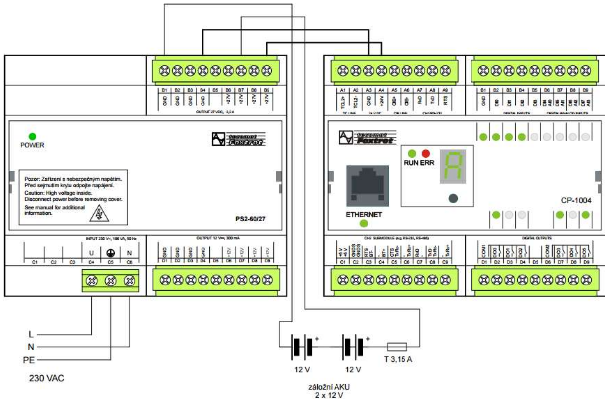
Obr. 3-14: Příklad zálohového napájení základního modelu CP-1004 [17]
