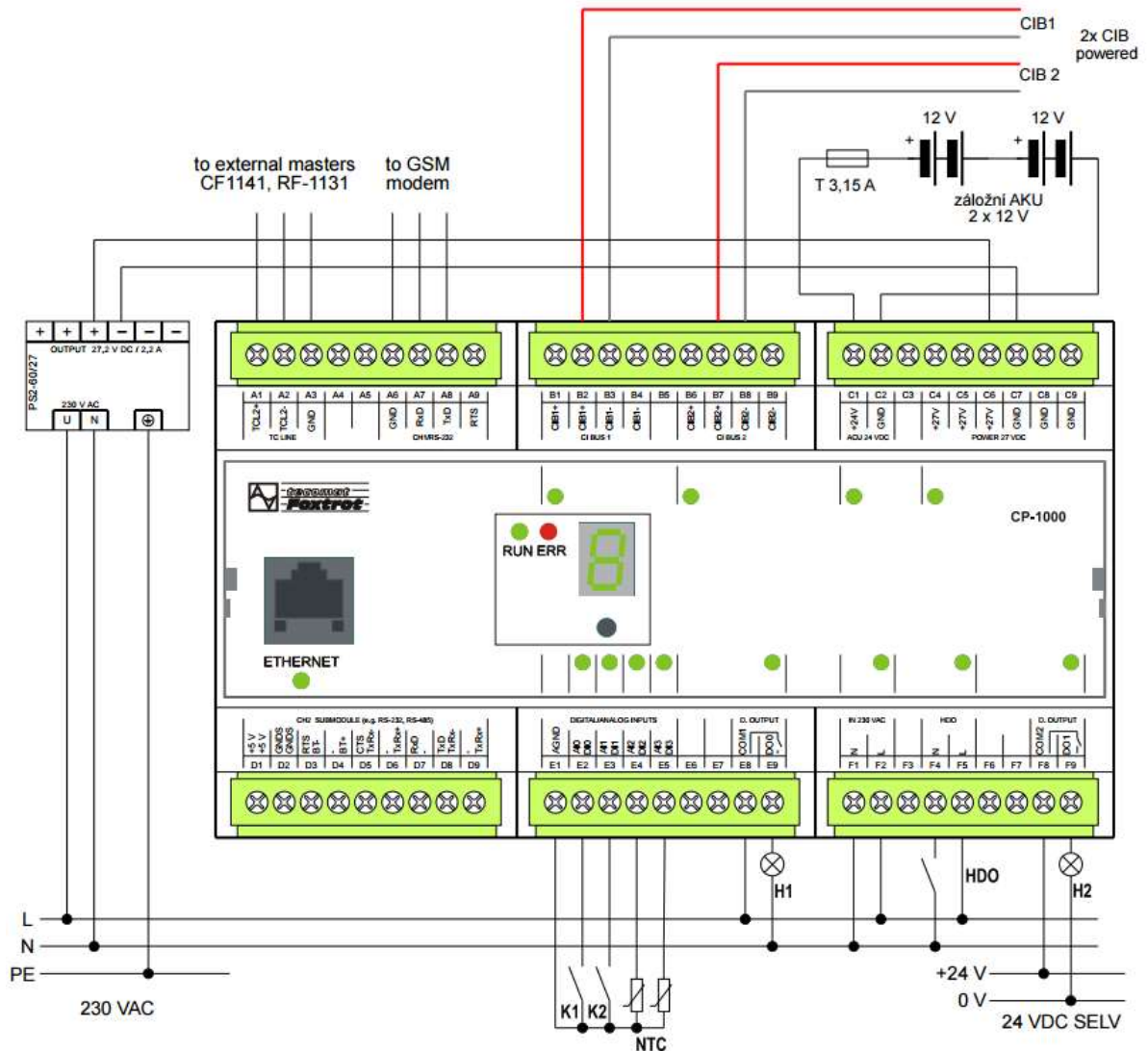
Obr. 3-11: Základní jednotka CP-1000 [21]
