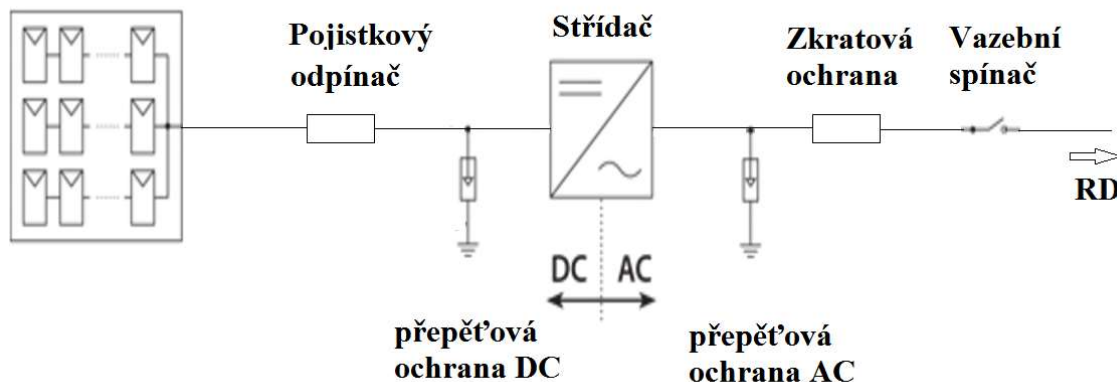
Obr. 5-4: Blokové schéma fotovoltaické elektrárny
