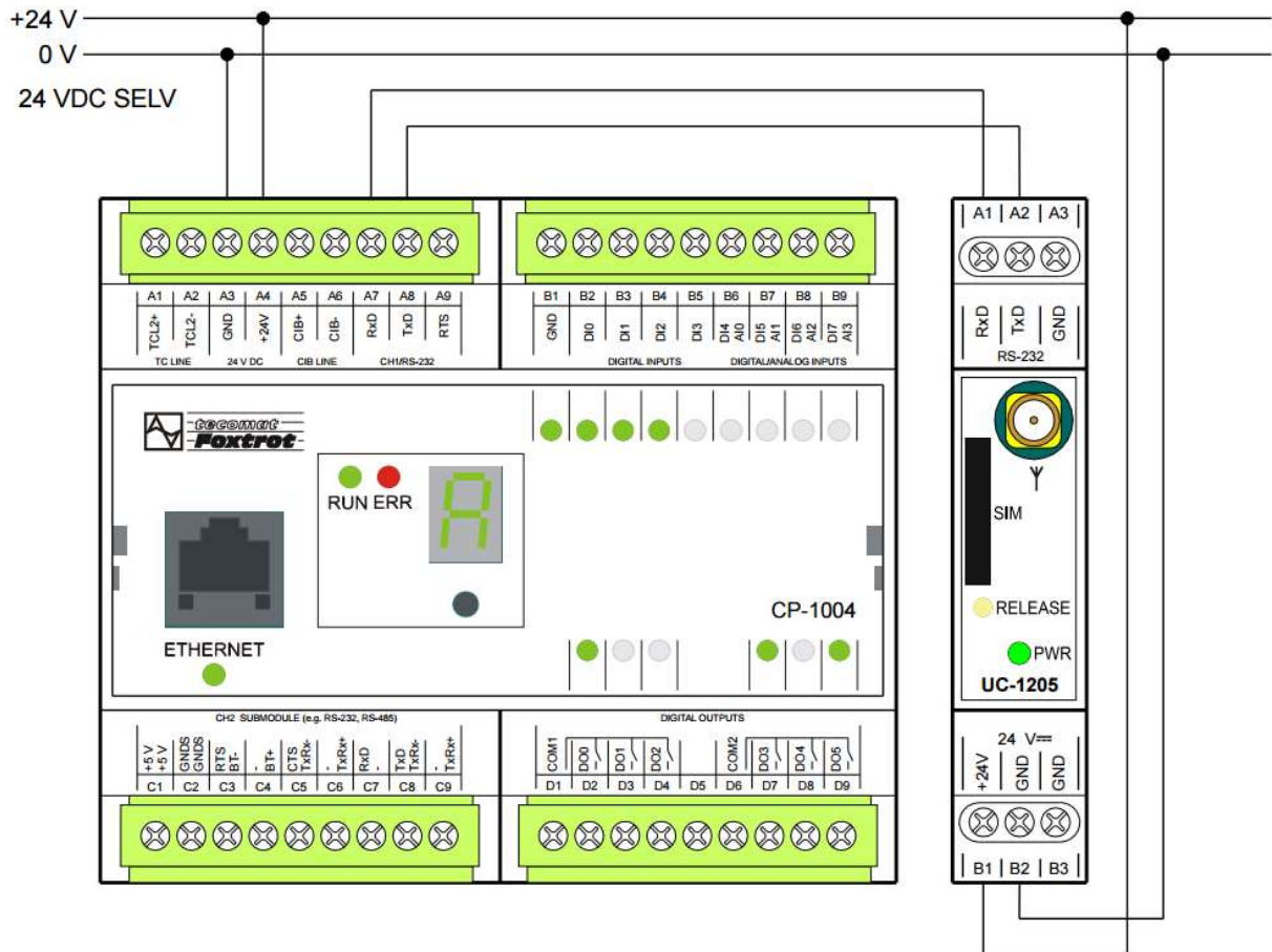
Obr. 3-16: Zapojení GSM modulu [17]
