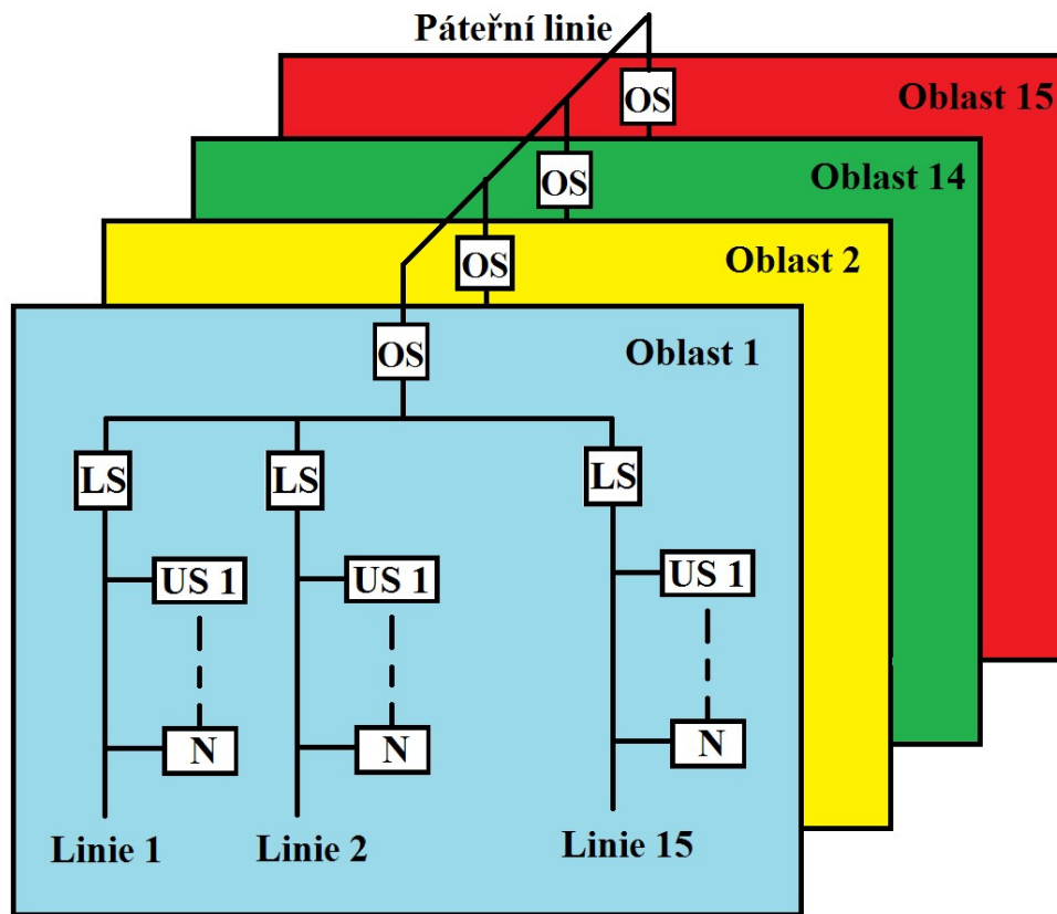
Obr. 3-6: Topologie systému KNX [9]
