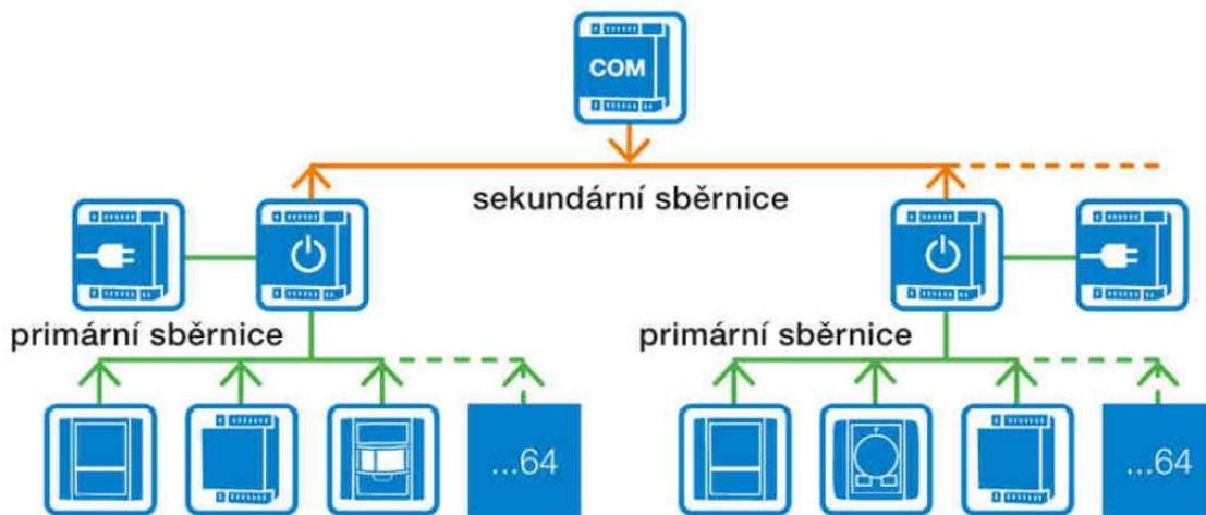
Obr. 3-7: Topologie systému Ego-n [11]
