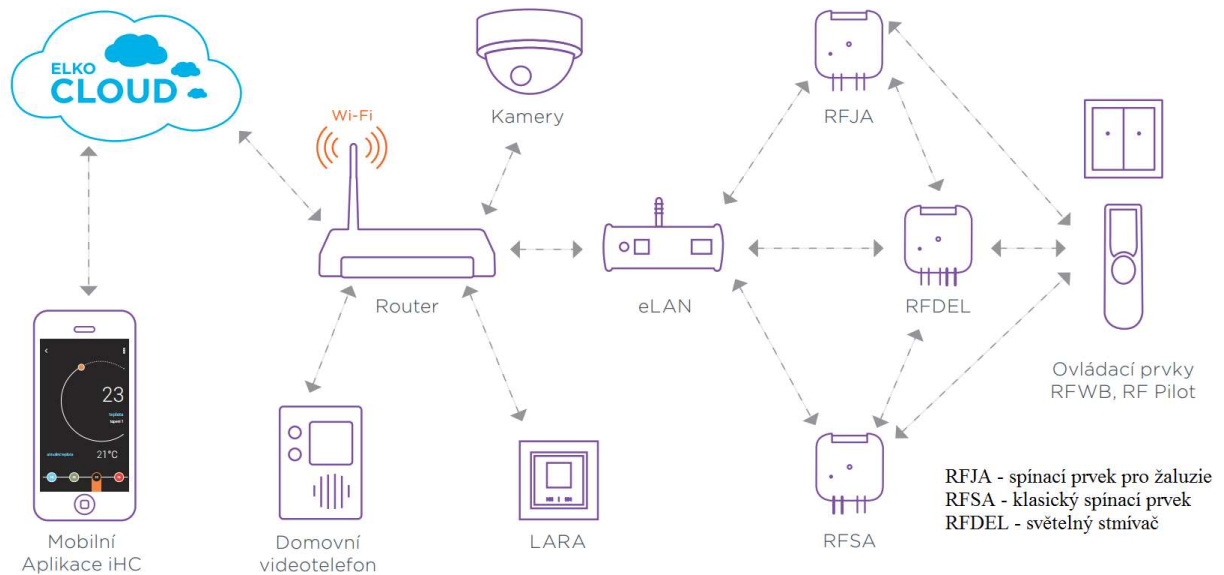
Obr. 3-8: Funkční diagram iNELS RF Control [13]
