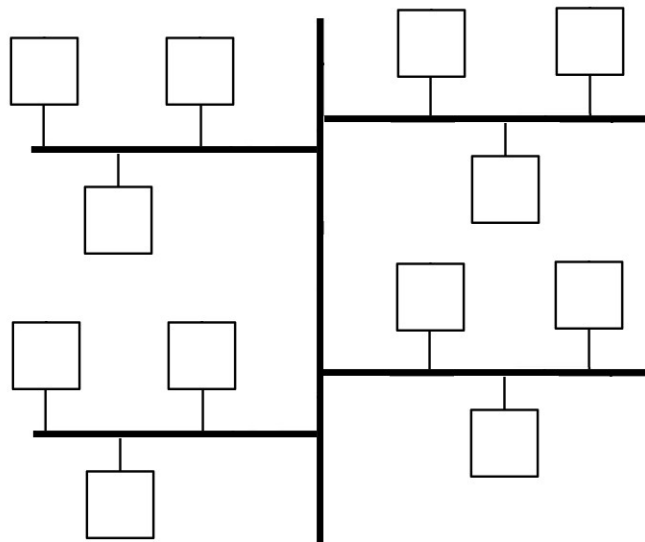
Obr. 3-5: Stromová struktura sběrnice [5]
