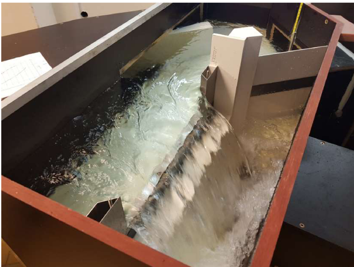
Obr. 26) Měření přepadu pouze přes tabulový uzávěr
