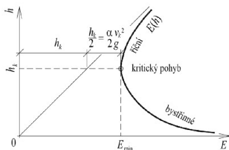
Obr. 1) Energetická výška průřezu [2]
