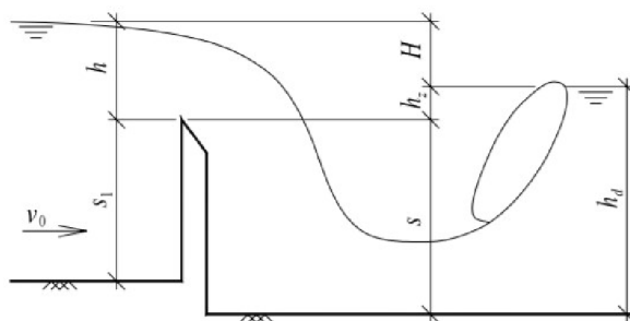
Obr. 5) Dokonalý přepad [1]
