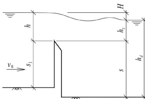
Obr. 6) Nedokonalý přepad [1]
