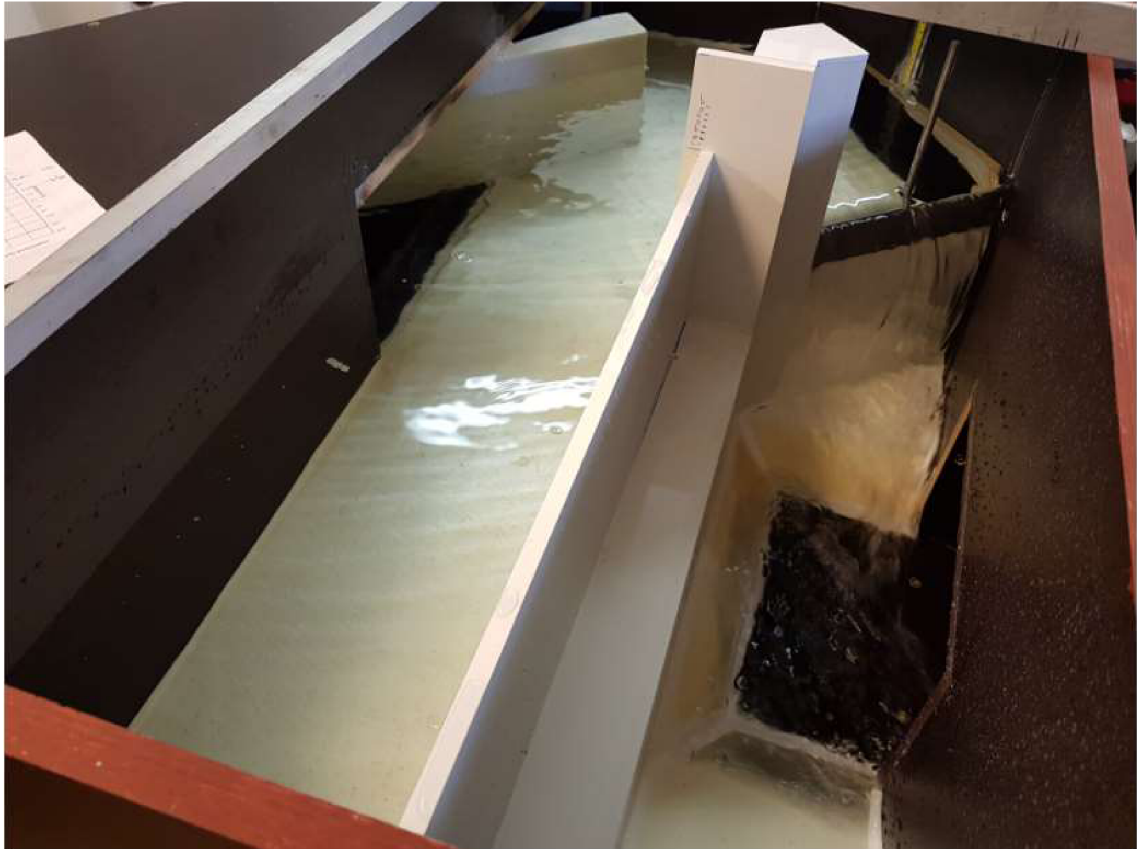
Obr. 25) Měření s podmínkou přepadu pouze přes pevné stavidlo
