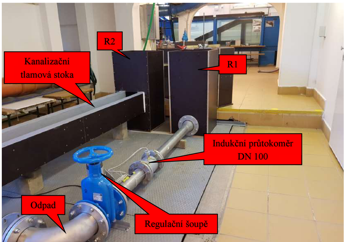
Obr. 20) Protiproudni pohled na nádrže R1 a R2 a odtoků z nich
