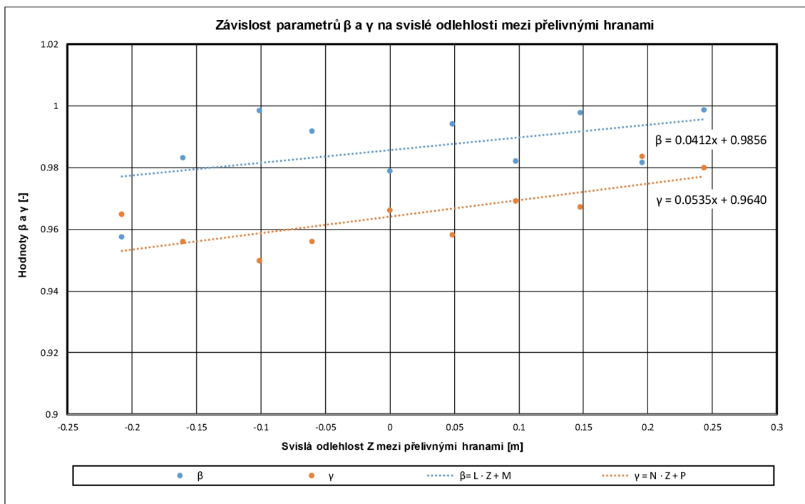
Graf 9) Nalezení lineárních funkcí pro hodnoty \beta a \gamma
