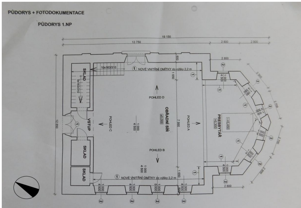
33. Kaple s. Alžběty v Buchlovicích – půdorys
