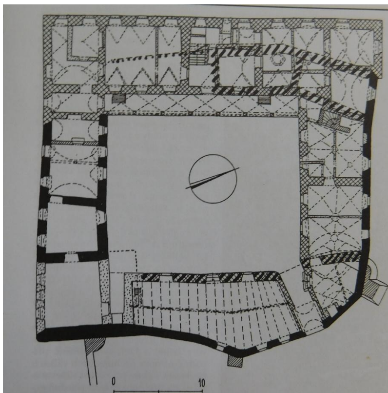
45. Zámek v Krakovci-Laškově – půdorys zámku, mřížkované zdivo bylo vystavěno za Zástřizlů mezi lety 1611 - 1614
